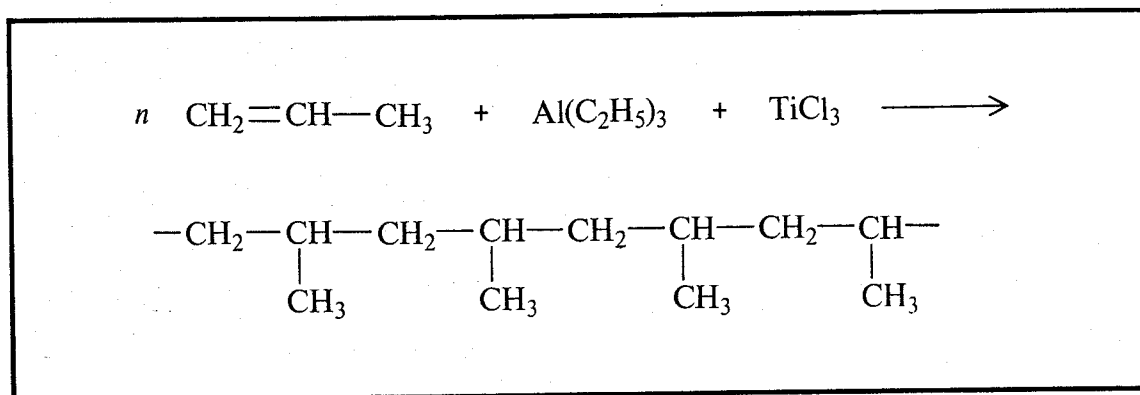
Fig.82 In presenza di catalizzatori simili ai precedenti (ad esempio costituiti da alluminotrietile e tricloruro di titanio) il propilene si converte in un prodotto che non era mai stato ottenuto per altra via: il polipropilene isotattico, un polimero che fonde a 175 °C.
