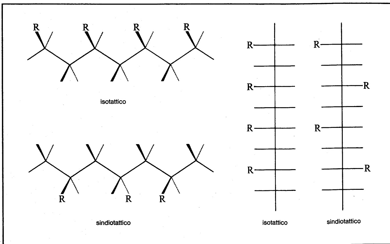
Fig.86 Le relazioni configurazionali esistenti nel polimero vengono rese più evidenti quando la catena polimerica viene stesa a zig-zag su un piano o viene rappresentata in proiezione di Fischer. Nei polimeri isotattici il sostituito R si trova sempre dalla stessa parte, nei polimeri sindiotattici si trova invece una volta da una parte, una volta dall'altra.
