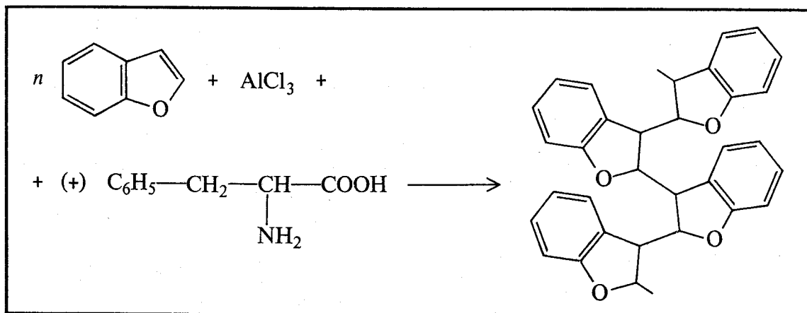
Fig.118 Polimerizzazione asimmetrica del benzofurano. Per azione del catalizzatore asimmetrico formato dal tricloruro di alluminio e da un amminoacido otticamente attivo, la fenilalanina, il benzofurano si converte in un polimero dotato di un alto potere rotatorio.
