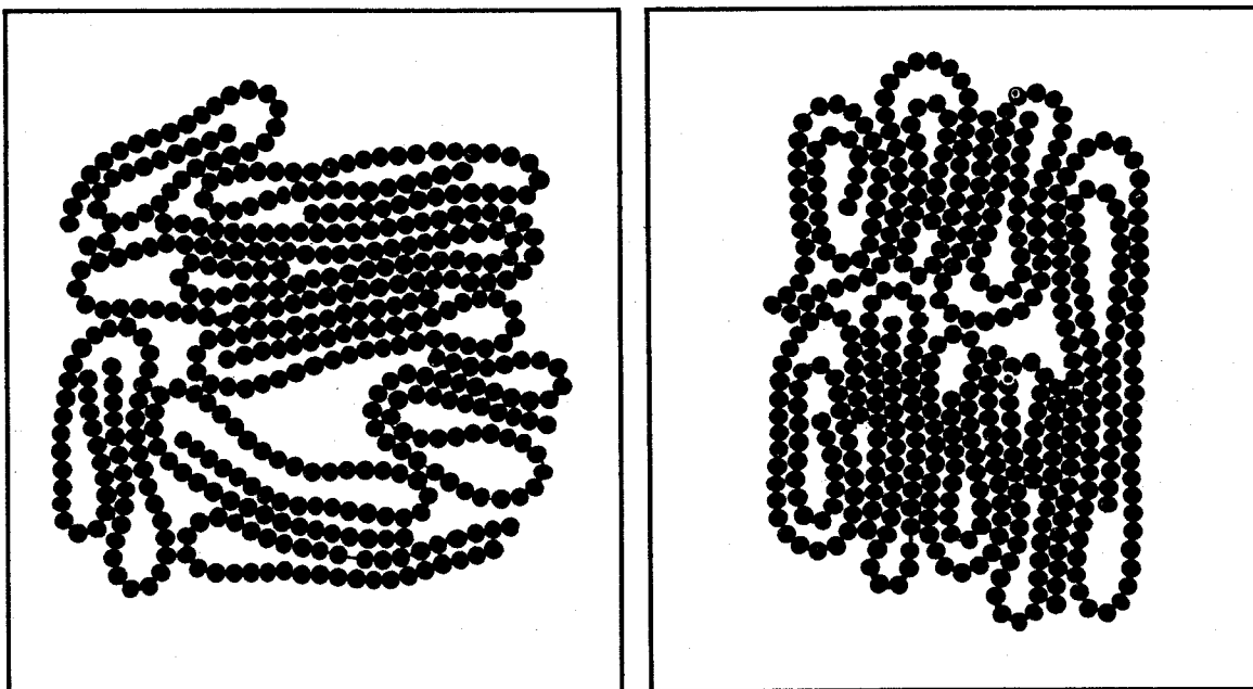
Fig.93 Nelle lamine parzialmente cristalline si hanno delle regioni ordinate in cui le macromolecole sono parallele fra loro ed altre zone disordinate. Quando la lamina viene stirata gli assi dei vari cristalli si dispongono lungo la direzione di stiro e risultano paralleli. Con questo processo le proprietà meccaniche del polimero migliorano notevolmente.
