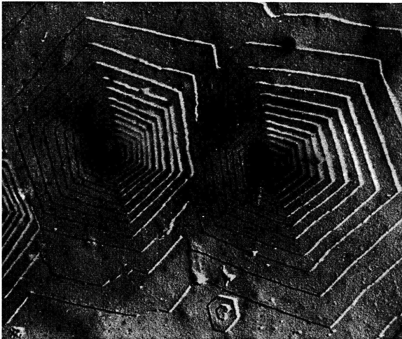
Fig.92 Fotografia al microscopio elettronico di un monocristallo di polioossimetilene. Contrariamente a quanto si potrebbe supporre, le macromolecole sono disposte in modo perpendicolare al piano di massima estensione del cristallo (foto General Electric Company ).
