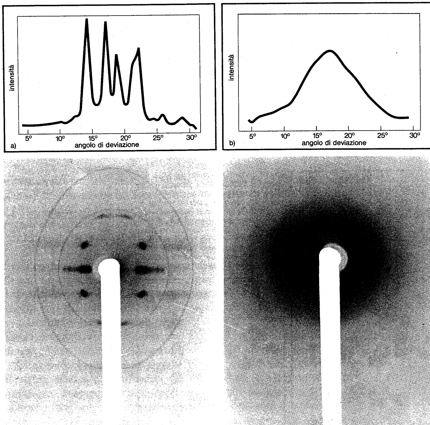
Fig.83 Come si presentano gli spettri di diffrazione dei raggi X del polipropilene isotattico cristallino (a sinistra) e di un polipropilene amorfo. La registrazione degli spettri viene ottenuta con un contatore Geiger (in alto) oppure con tecniche fotografiche. La cristallinità del polimero è rivelata dalla presenza di picchi e di macchie in posizioni ben definite.
