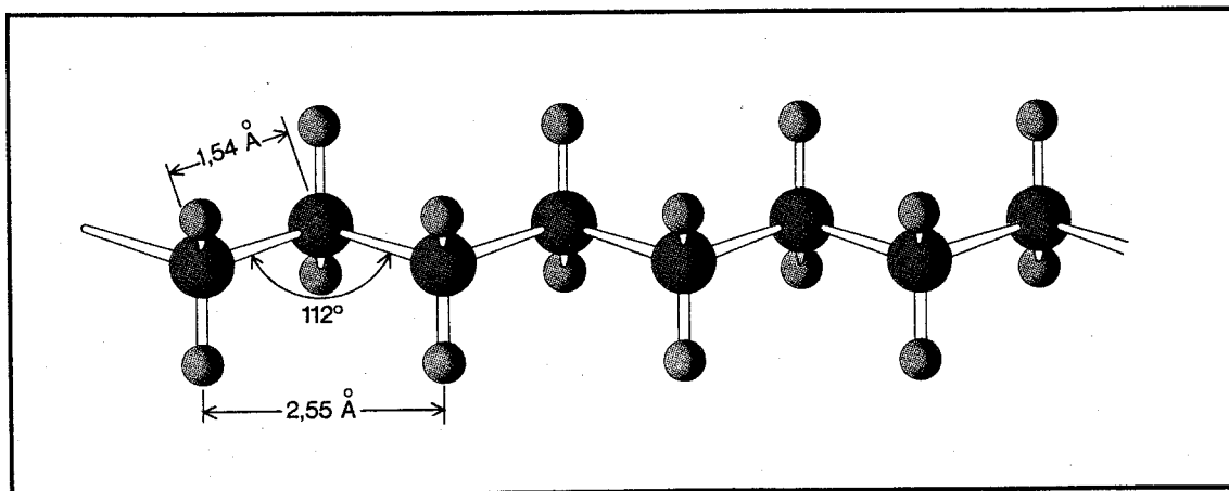
Fig.84 Conformazione della catena del polietilene allo stato cristallino. Gli angoli di rotazione interna sono di 180^\circ (conformazione anti ). Il periodo di ripetizione, 2,55 Å, concorda con quello calcolato usando i normali valori della lunghezza e dell'angolo di legame.
