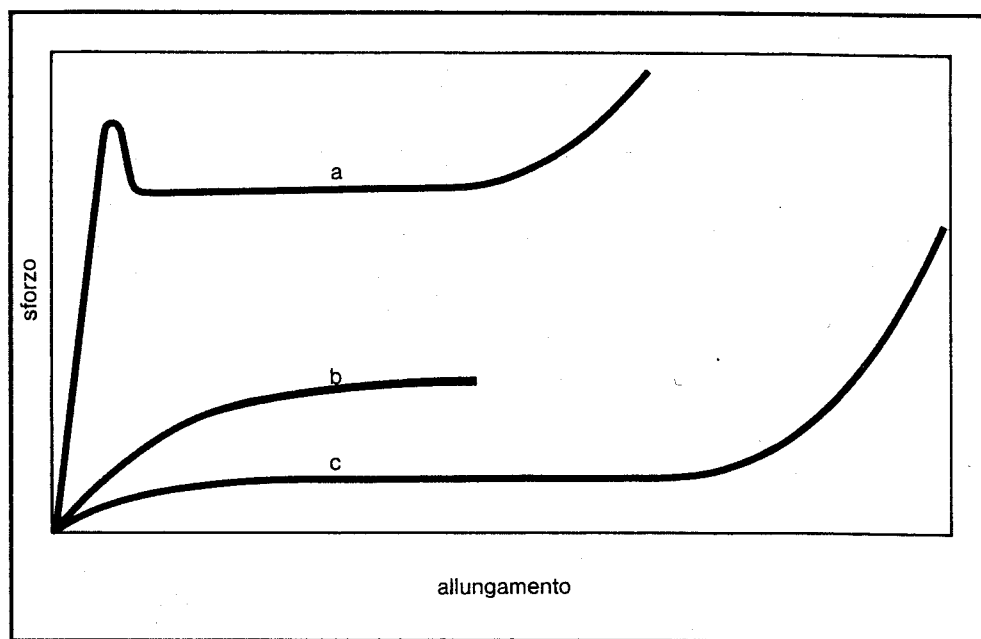
Fig.94 Le proprietà meccaniche dei diversi tipi di polimero sono illustrate da questo diagramma sforzo-allungamento. Viene indicato il comportamento tipico di un polimero cristallino (a), di un polimero amorfo (b) e di una gomma (c). Il massimo carico di rottura si osserva nei prodotti cristallini, mentre il massimo allungamento si verifica nelle gomme.
