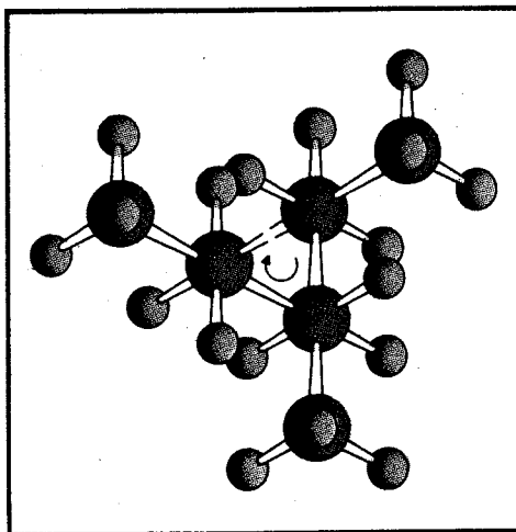
Fig.85 Conformazione ad elica ternaria del polipropilene isotattico allo stato cristallino. Gli angoli di rotazione interna sono alternatamente di 180^\circ e 60^\circ ; la catena può essere descritta come una successione di conformazioni T, G, T, G , ecc. ( T = trans o anti , G = gauche o sghemba ). I gruppi metilici sono disposti all'esterno in modo da rendere minima l'interazione col resto della catena.
