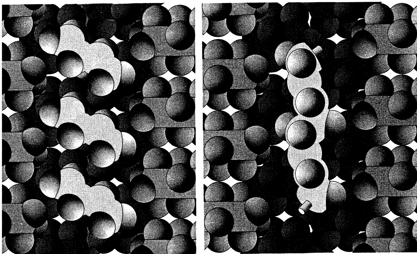
Fig.121 A sinistra, cella cristallina del peridrotifenilene. Sono visibili le dimensioni di ingombro delle molecole, come si ottengono usando i modelli molecolari a sfera. Agli spigoli della cella cristallina si può vedere una zona vuota, in cui si dispongono le molecole ospiti. Qui sopra, struttura del composto di inclusione peridrotifenilene-butadiene (a sinistra) e peridrotifenilene-polibutadiene. In basso schema della polimerizzazione. La struttura del polimero è 1,4- trans . La sintesi asimmetrica descritta nel testo è stata effettuata sul pentadiene, ultima formula in basso. Il corrispondente polimero, del tipo 1,4- trans isotattico, contiene un atomo di carbonio asimmetrico in ogni unità monomerica.
