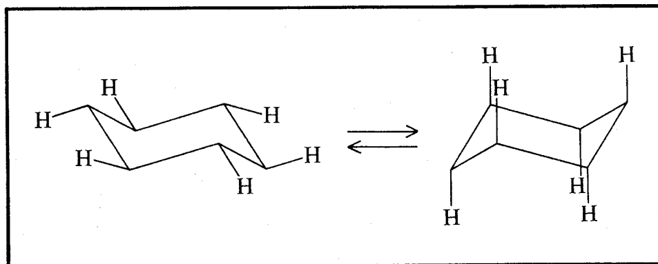
Fig.37 Le forme a sedia e a barca del cicloesano (in alto). Nella realtà il cicloesano possiede una struttura molto vicina a quella teorica a sedia, con angoli di valenza quasi esattamente tetraedrici ( 111,5^\circ contro 109,5^\circ ) e angoli di rotazione di 55^\circ , molto prossimi a quelli teorici ( 60^\circ ). La forma a barca non è presente in concentrazioni apprezzabili nel cicloesano, ma esiste in alcuni composti più complessi, ad esempio nella canfora (si veda la Fig. 28). Al centro, i due tipi di idrogeni presenti nella forma a sedia del cicloesano, quelli assiali e quelli equatoriali. In basso: l'equilibrio conformazionale del metilcicloesano è spostato di molto verso la forma col metile equatoriale (nel rapporto 95 : 5). A sua volta il terziario -butilcicloesano esiste solo in forma equatoriale, a causa del maggior ingombro del sostituyente.
