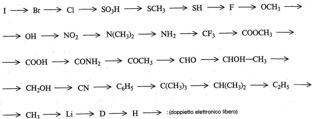
Fig.123 Priorità di alcuni fra i più comuni sostituenti secondo la nomenclatura di Cahn, Ingold e Prelog.
