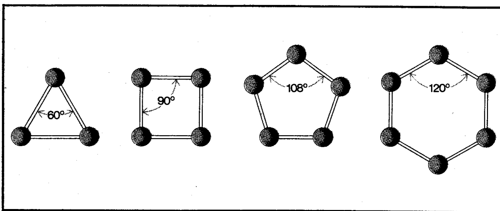
Fig.10 Struttura degli idrocarburi ciclici secondo la teoria di Baeyer basata sulla planarità della struttura e sulla tensione degli angoli di valenza (gli atomi di idrogeno non sono indicati). Anche se può spiegare alcuni fatti sperimentali, la teoria di Baeyer non è fisicamente accettabile. L'indagine moderna ha invece confermato l'ipotesi di Sachse sulla non planarità della struttura del cicloesano.
