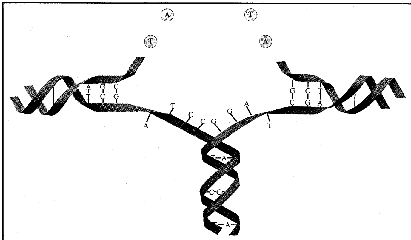
Fig.105 Schema formale di duplicazione del DNA: la doppia elica si apre e su ciascuna matrice si riproduce una catena complementare, esattamente identica a quella primitiva.
