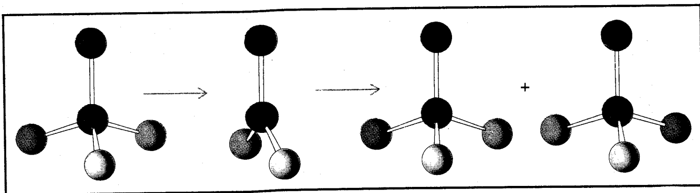
Fig.64 La reazione di sostituzione AX + Y^- = AY + X^- viene chiamata S_N1 quando segue una equazione cinetica del primo ordine ( v = K[A] ). La specie attivata è costituita da uno ione carbonio positivo prodotto dall'eliminazione di X^- . La struttura pianosimmetrica dello ione carbonio fa in modo che l'attacco del reagente Y^- avvenga con uguale probabilità sulle due facce opposte, con formazione di un ugual numero di molecole antipode.
