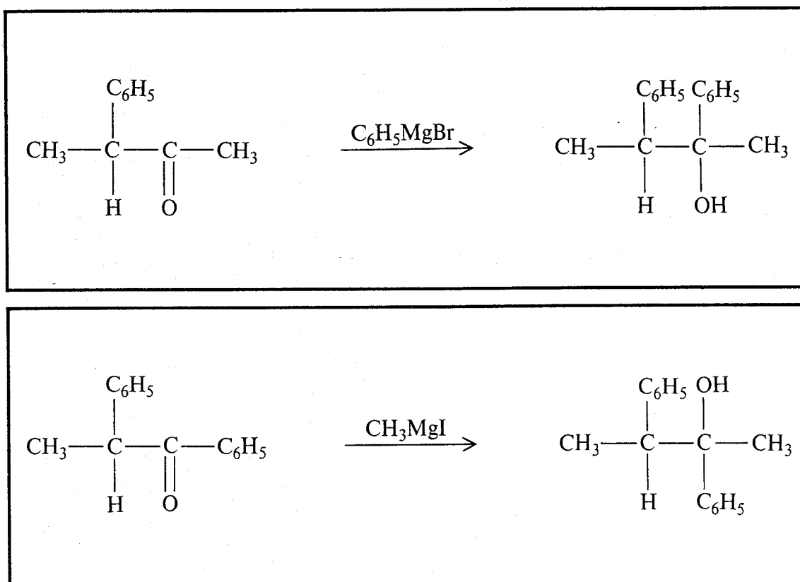
Fig.74 La reazione di un chetone con un composto organico del magnesio conduce alla formazione di un alcool terziario che contiene nella molecola anche il residuo organico in origine legato al magnesio. L'inversione dell'ordine di introduzione dei diversi radicali organici porta a due diversi diastereoisomeri. L'asimmetria del chetone esercita una induzione asimmetrica sulla reazione, favorendo la formazione di particolari stereoisomeri.
