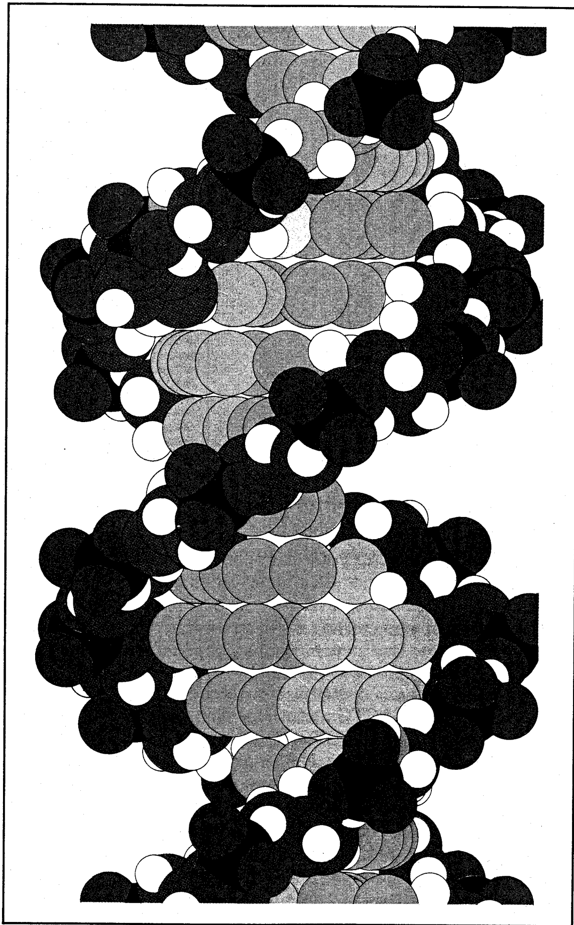
Fig.104 La doppia elica del DNA determinata per mezzo dell'analisi cristallografica.
