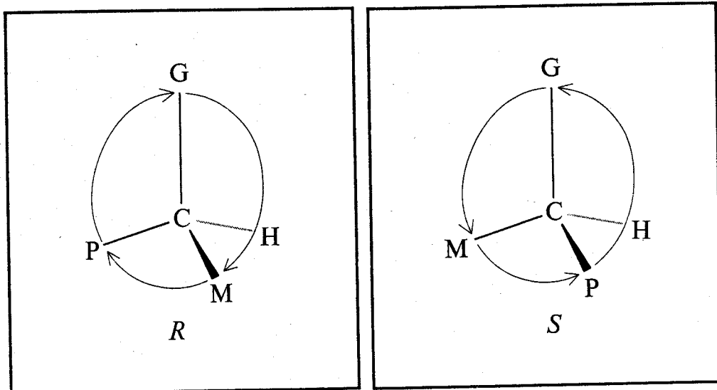
Fig.124 Modo di osservazione di un atomo tetraedrico e assegnazione della sua configurazione assoluta.
