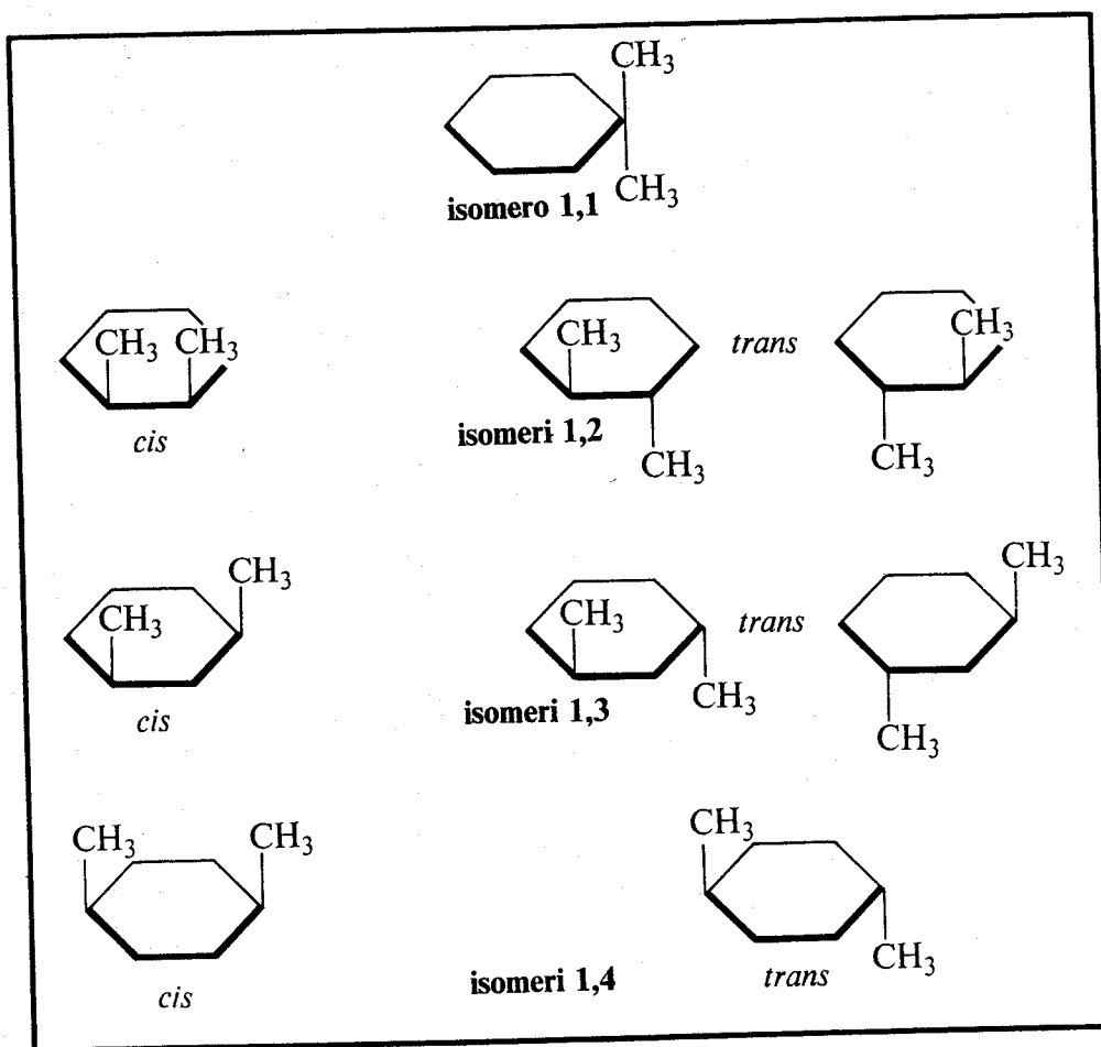
Fig.31 Gli isomeri possibili del dimetilcicloesano sono sette se si considera come un unico composto ogni coppia di antipodi (quelle dell'1,2- e dell'1,3- trans -dimetilcicloesano), oppure nove se si contano anche gli antipodi configurazionali. Per determinare il numero degli isomeri l'anello del cicloesano può essere considerato un esagono piano.
