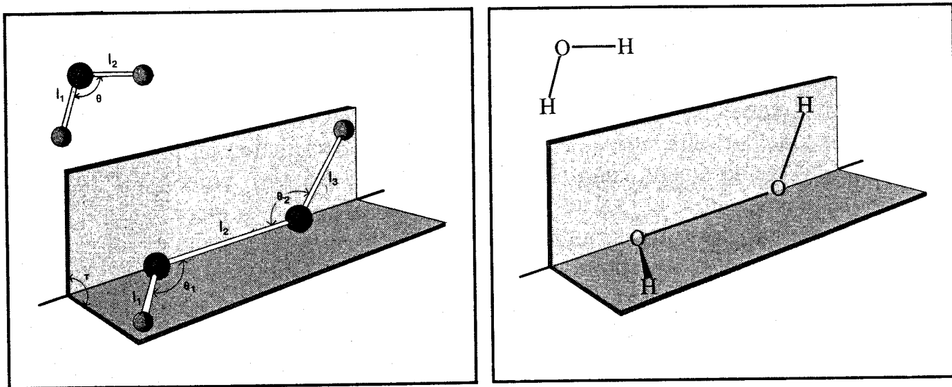
Fig.32 Parametri geometrici in un sistema di tre punti e di quattro punti non coplanari. A destra, struttura dell'acqua H_2O e dell'acqua ossigenata H_2O_2 . Quest'ultima rappresenta la molecola piú semplice su cui si può compiere un'analisi conformazionale. L'angolo di rotazione nella conformazione stabile dell'acqua ossigenata è prossimo a 90^\circ .
