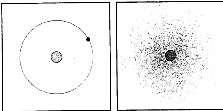
Fig.15 Secondo la teoria di Bohr l'elettrone dell'atomo di idrogeno allo stato fondamentale ruota attorno al nucleo a distanza fissa, uguale a 0,53 \text{ \AA} . Secondo la teoria quantomeccanica si può parlare soltanto della probabilità di trovare l'elettrone ad una certa distanza dal nucleo. Tale probabilità è massima su una sfera di raggio uguale a quello dell'orbita di Bohr, ma ha un valore finito anche a distanze maggiori e minori dal nucleo.
