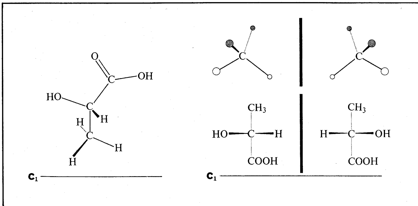
Fig.51 Una delle conformazioni dell'acido lattico in cui non esiste alcun elemento di simmetria (gruppo C_1 ). Anche se si facessero ruotare i vari gruppi attorno ai legami che li uniscono all'atomo centrale, la struttura sarebbe sempre asimmetrica: quattro sfere diverse poste ai vertici di un tetraedro costituiscono infatti un sistema asimmetrico. A destra in basso, le formule dei due antipodi dell'acido lattico. L'atomo centrale legato a quattro sostituenti diversi ( -H , -OH , -CH_3 , -COOH ) è detto atomo di carbonio asimmetrico.
