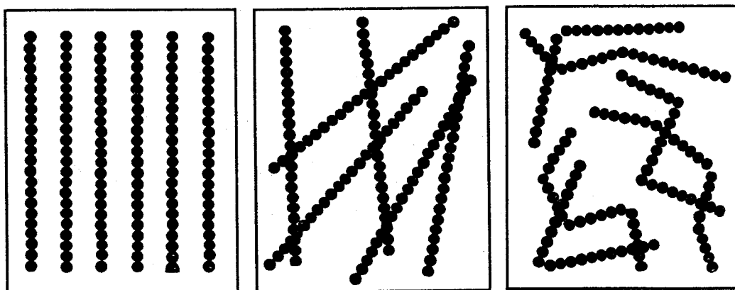
Fig.106 I due stadi di cui è idealmente formato il processo di fusione di un cristallo. Si può pensare che le molecole dapprima siano disposte nel cristallo in modo regolare e poi si allontanino e cambino l'orientamento reciproco rimanendo ancora rigide. Successivamente esse assumono forme diverse secondo le regole statistiche già ricordate.
