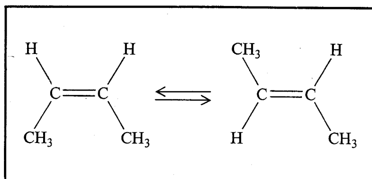
Fig.30 In alto: il primo composto si differenzia strutturalmente dagli altri, mentre il secondo e il terzo sono stereoisomeri, ossia sono diversi fra loro solo per quanto riguarda la disposizione delle valenze nello spazio. L'isomeria cis-trans esiste anche nei composti con due o più doppi legami. Al centro l'acido cis , trans -sorbico e l'acido trans , trans -sorbico. I due composti indicati in basso, il cis - e il trans -2-butene, sono stabili, ma in particolari condizioni possono convertirsi facilmente l'uno nell'altro.
