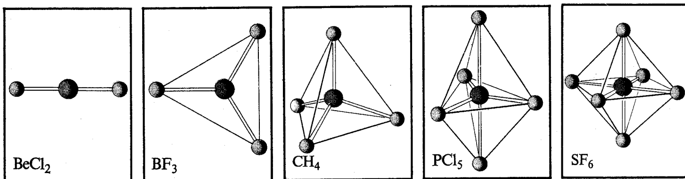
Fig.25 Quando l'atomo centrale di una molecola è circondato da due, tre, quattro, cinque o sei atomi e non possiede doppietti elettronici liberi, la forma della molecola è rispettivamente lineare, triangolare piana, tetraedrica, a bipiramide trigonale ed ottaedrica, a meno di deformazioni dovute alla diversa natura degli atomi.
