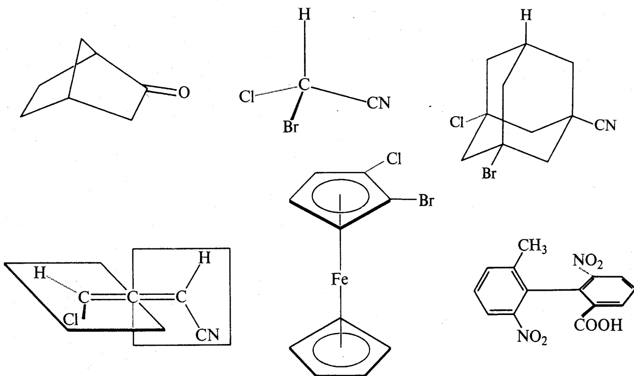
Fig.47 Le molecole asimmetriche non contengono alcun elemento di simmetria: esse appartengono secondo la nomenclatura di Schoenflies (si veda l'Appendice III) al gruppo C_1 . Da sinistra a destra e dall'alto verso il basso, una serie di strutture asimmetriche rigide; la nor -canfora, il clorobromoacetone, il clorobromoadamantilcianuro, l'1-cian,3-cloroallene, l'1-cloro,2-bromoferrocene, il 2,2'-dinitro,6-metil,6'-carbossidifenile.
