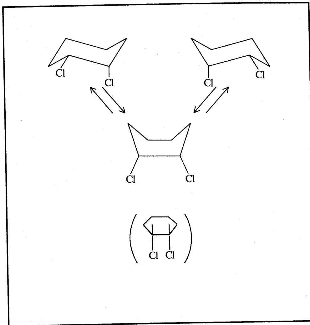
Fig.54 Il cis -1,2-diclorocicloesano esiste in due conformazioni stabili asimmetriche e interconvertibili tra loro. In questo caso non esiste alcuna conformazione non-dissimmetrica stabile. Tuttavia si può pensare a uno stato di transizione (instabile) non-dissimmetrico.
