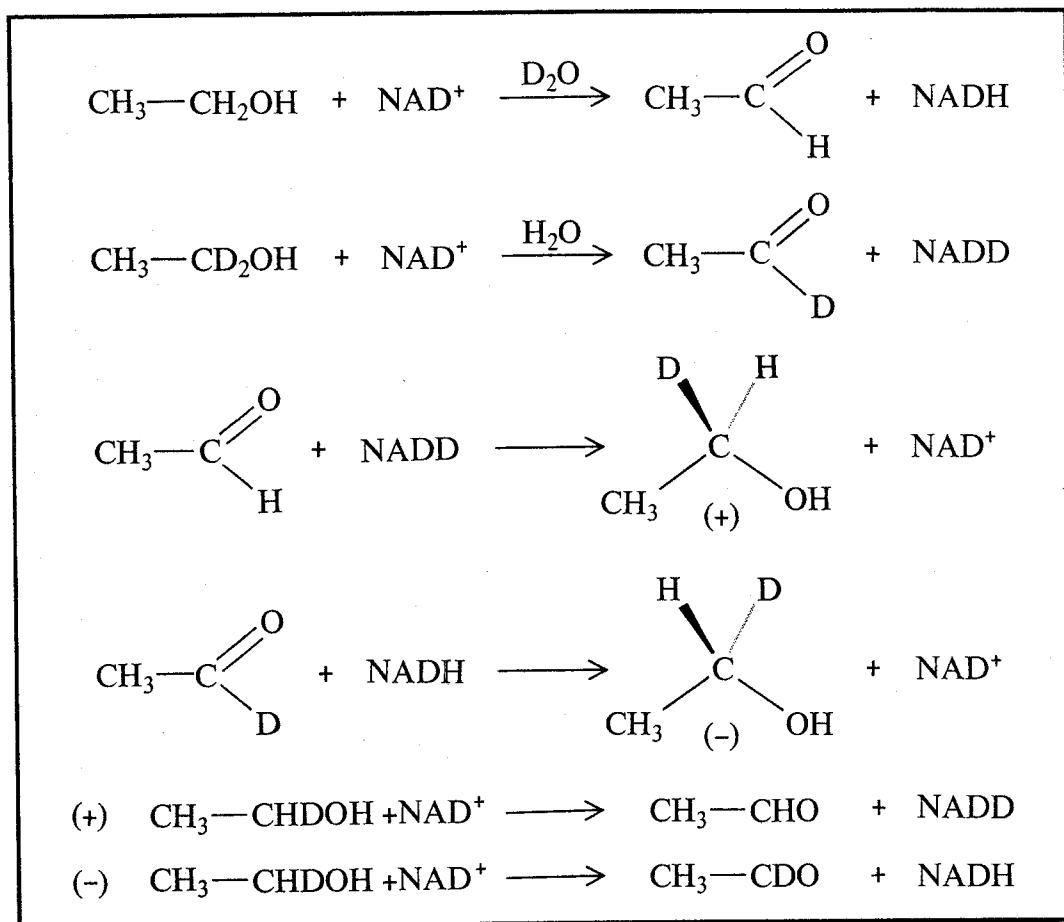
Fig.112 Alcuni aspetti stereochimici delle reazioni enzimatiche sono chiaramente illustrati nel processo ossidoriduttivo realizzato da Westheimer sull'alcool etilico. 1) Ossidazione dell'alcool in acqua pesante: non si ha incorporazione di deuterio. 2) Ossidazione dell'alcool deuterato: si forma l'aldeide deuterata e il coenzima ridotto deuterato. 3) Riduzione dell'aldeide non deuterata col coenzima deuterato: si ottiene alcool monodeuterato positivo. 4) Riduzione dell'aldeide deuterata col coenzima non deuterato: si ottiene l'alcool monodeuterato negativo. 5) Ossidazione dell'alcool deuterato positivo: si ottiene l'aldeide non deuterata. 6) Ossidazione dell'alcool deuterato negativo: si ottiene l'aldeide deuterata. Il coenzima agisce in modo totalmente stereospecifico, cedendo o togliendo un atomo di idrogeno (o di deuterio) sempre nella stessa posizione.
