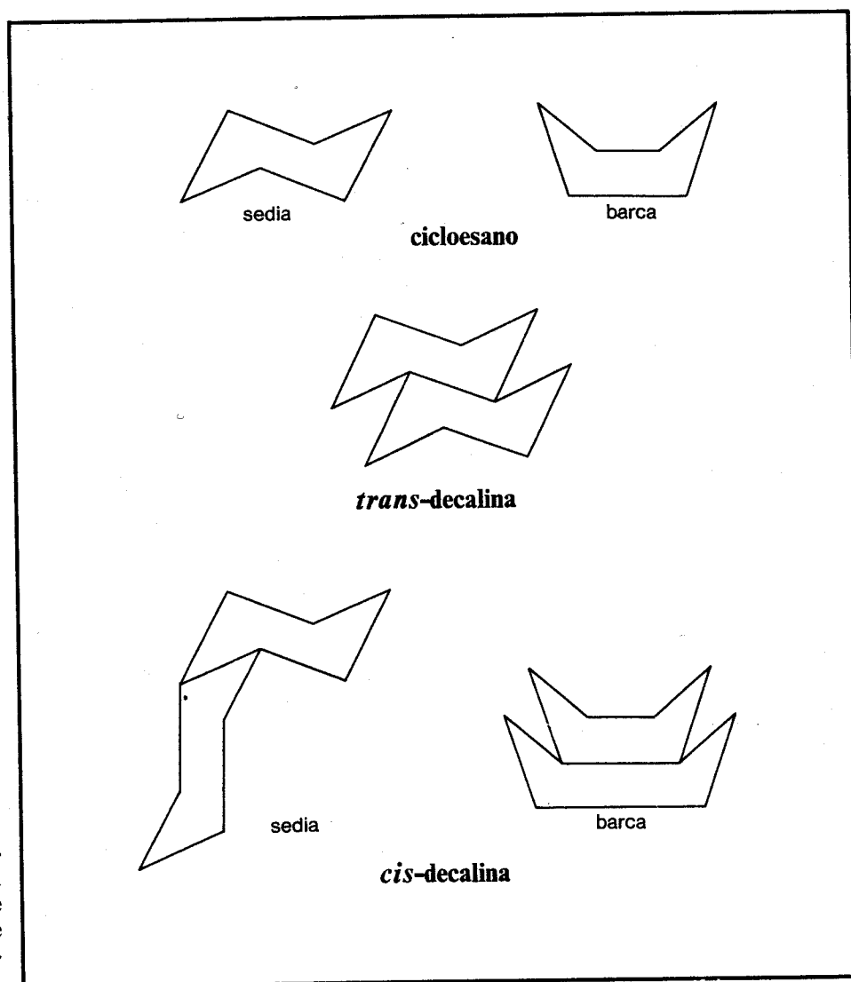
Fig.11 Struttura degli idrocarburi ciclici secondo la teoria di Sachse. Dall'alto forma a sedia e a barca del cicloesano, forma a sedia della trans -decalina, forme a sedia e a barca della cis -decalina. L'indagine più recente ha dimostrato che la cis -decalina esiste nella forma a sedia (in basso a sinistra).
