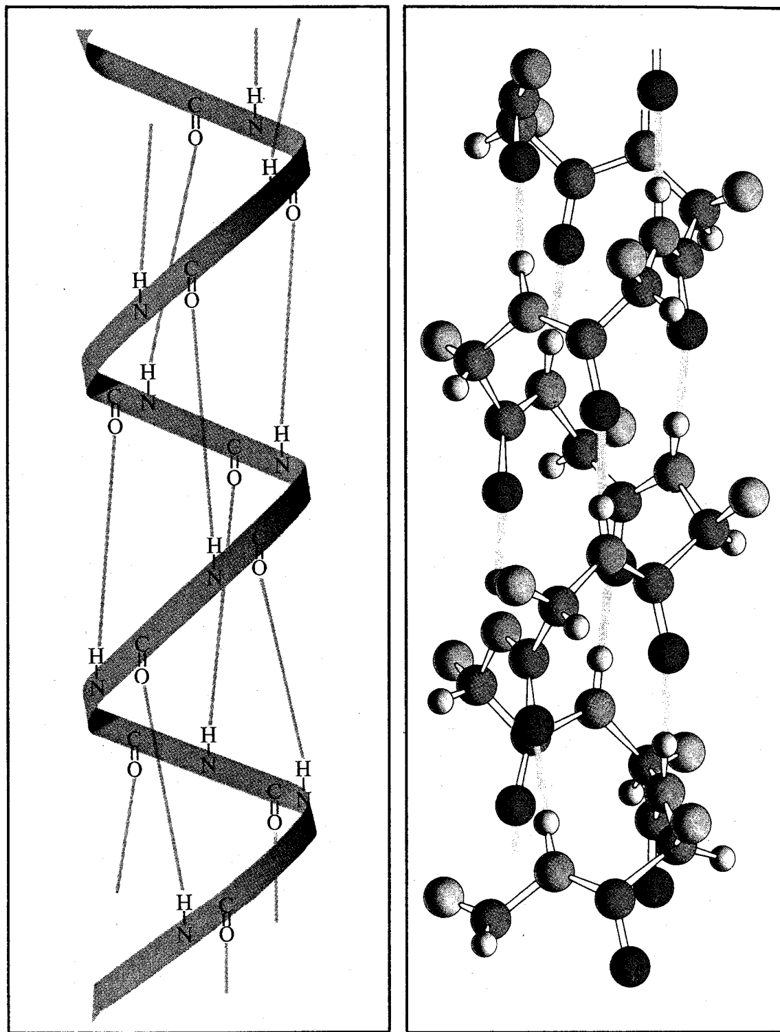
Fig.99 La conformazione più comune nelle catene polipeptidiche allo stato cristallino è l' \alpha -elica di Pauling. La sua stabilità è dovuta sia alla formazione di numerosi legami a idrogeno intramolecolari sia alla favorevole disposizione dei sostituenti laterali.
