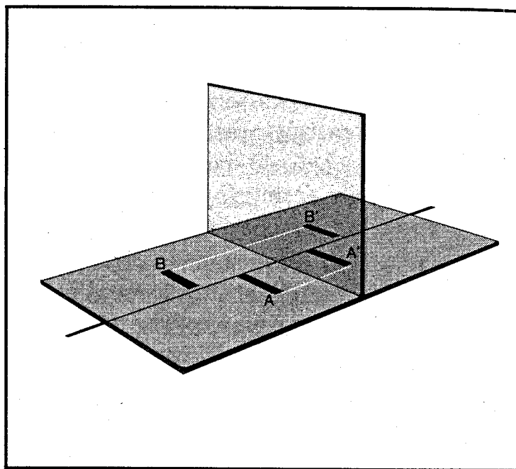
Fig.117 Oltre agli elementi di simmetria descritti nel IV capitolo, per i composti macromolecolari bisogna considerare anche i piani di simmetria con traslazione, caratterizzati da un'operazione di riflessione e da una di traslazione lungo un asse contenuto nel piano. Da sinistra, schemi di un piano di simmetria perpendicolare all'asse della catena polimerica, di un piano di simmetria contenente l'asse delle catene e di un piano di simmetria con traslazione contenente l'asse della catena.
