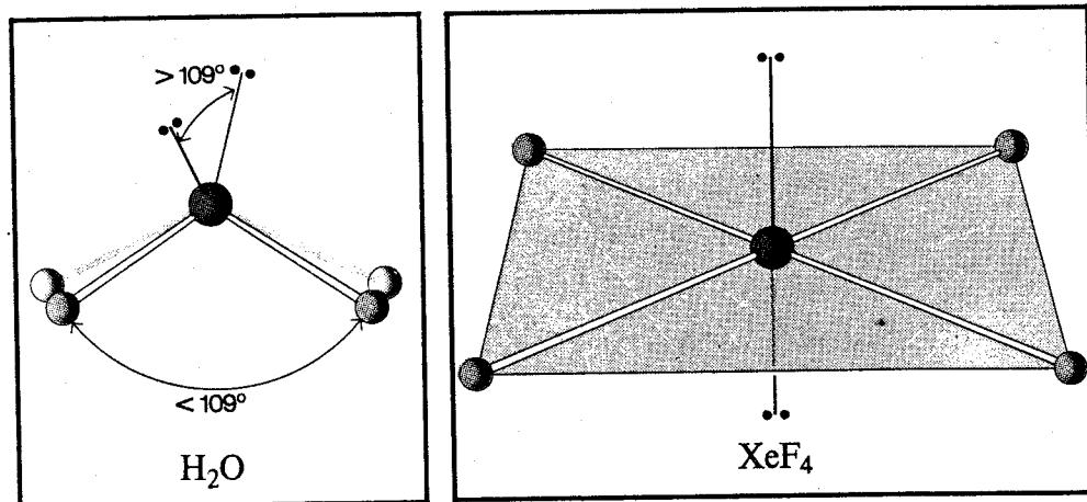
Fig.26 Se sono presenti dei doppietti elettronici liberi, questi tendono ad allontanarsi fra loro. Nella molecola dell'acqua questo fatto porta ad una deformazione dell'angolo di valenza che si stringe di circa 5^\circ rispetto al previsto. Nel tetrafluoruro di xenone, un composto dei gas nobili, i doppietti di elettroni si dispongono ai vertici opposti dell'ottaedro.
