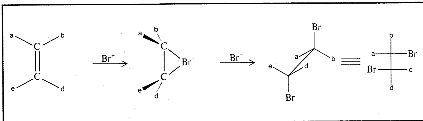
Fig.70 L'addizione di due atomi di bromo ad un'olefina avviene in due stadi. Dapprima si somma un catione \text{Br}^+ formando un composto ciclico a tre atomi detto ione bromonio. L'anione \text{Br}^- si addiziona poi dalla parte opposta del ciclo causando una inversione di configurazione del carbonio. La reazione complessiva decorre perciò con un meccanismo trans .
