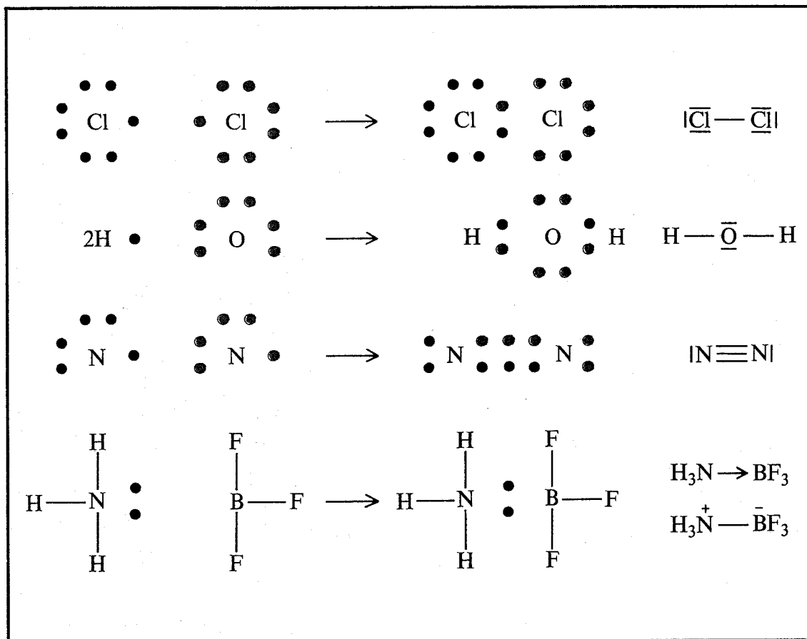
Fig.19 Alcuni esempi di molecole covalenti secondo la teoria di Lewis e Langmuir. Per facilitare la comprensione, gli elettroni appartenenti ad atomi diversi vengono disegnati in modo differente. A destra sono indicate le formule simboliche più usate: a ciascun trattino corrispondono due elettroni. Il legame covalente è formato da una o più coppie di elettroni messe in comune dai due atomi (si vedano le molecole del cloro \text{Cl}_2 , dell'acqua \text{H}_2\text{O} e dell'azoto \text{N}_2 ). Nel composto di addizione fra l'ammoniaca e il trifluoruro di boro il legame è di tipo dativo poiché i due elettroni provengono entrambi dall'atomo di azoto. Il legame dativo viene indicato con una freccia oppure con un trattino e coi segni + e - posti rispettivamente sull'atomo che dona gli elettroni e su quello che li riceve.
