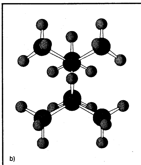
Fig.36 L'interazione fra atomi non direttamente legati, o interazione di Van der Waals, fra due gruppi metilici disposti come è indicato nella formula a1 dà alla molecola del 2,4-dimetilpentano un'energia troppo elevata. Per rotazione attorno ad un legame, la molecola si trasforma nella conformazione più stabile a2. Per il 2,2,4-trimetilpentano o iso -ottano non esiste alcuna conformazione sfalsata a bassa energia. La forma più stabile è quella con i due metili in basso eclissati rispetto ai due atomi di idrogeno centrali (b). Nel 2,2,4,4-tetrametilpentano la presenza di un ulteriore metile rende la molecola eccessivamente compressa: un'opportuna deformazione dell'angolo di valenza fa sì che i due atomi di carbonio quaternari si allontanino fra loro (c).
