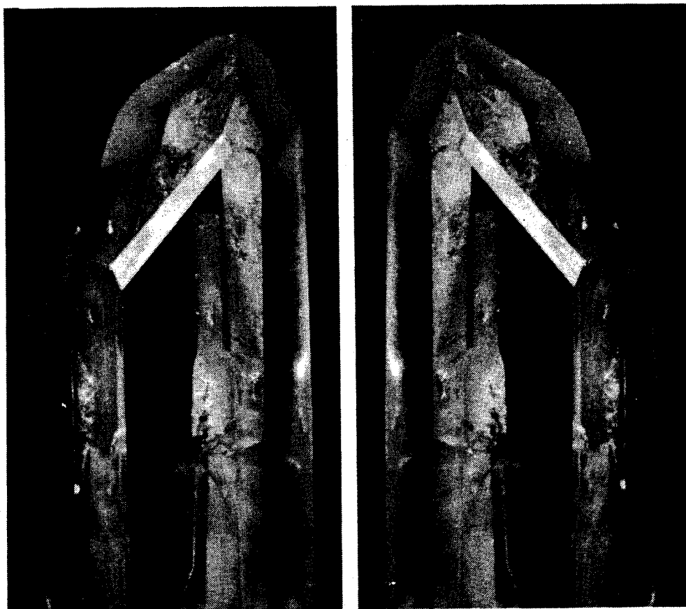
Fig.2 Due cristalli di quarzo enantiomorfi. Ciascuno è l'immagine speculare non sovrapponibile dell'altro. Per operare questo confronto sarebbe più opportuno esaminare dei cristalli ideali: anche in questi ultimi però la presenza di facce emiedriche orientate diversamente impedisce la sovrapposizione dei cristalli ( Fotografia Motto, Bottega delle pietre, Milano ).
