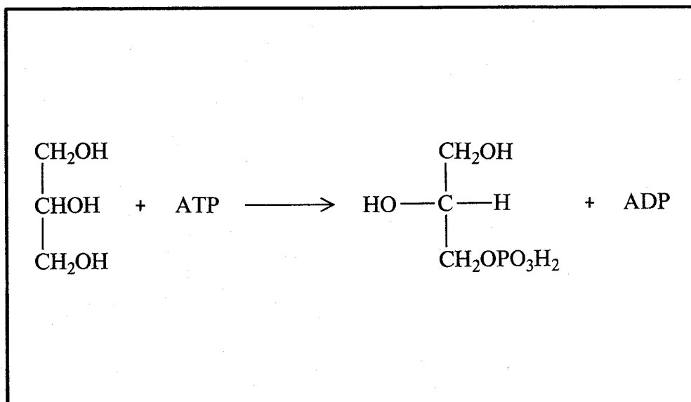
Fig.76 La fosfatazione della glicerina ad opera del coenzima ATP è un esempio di sintesi asimmetrica enzimatica. Benché i principi siano ancora quelli della chimica sintetica ordinaria, le reazioni enzimatiche si distinguono per una selettività sterica molto alta.
