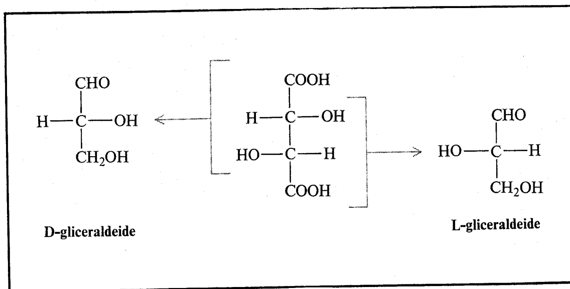
Fig.122 L'acido tartarico destrogiro, la cui formula è indicata al centro, è stato chiamato sia acido D-tartarico, sia acido L-tartarico. A seconda del metodo usato può essere correlato ad ambedue gli antipodi della gliceraldeide. Secondo la nuova nomenclatura l'antipodo qui rappresentato è chiamato, in modo completamente inequivocabile, R,R .
