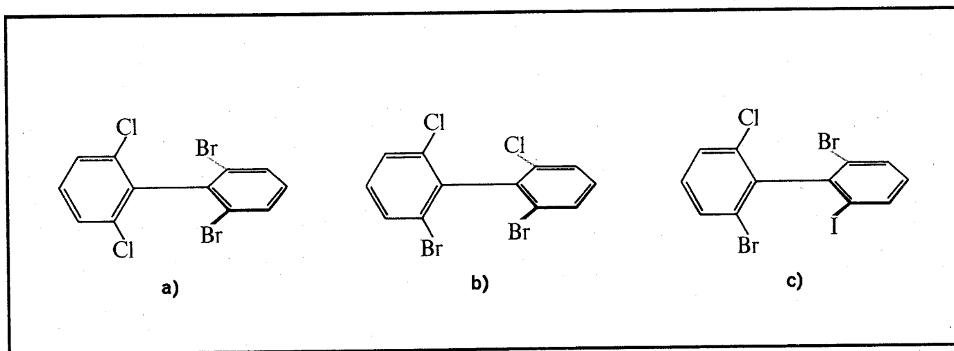
Fig.57 Tre esempi di derivati del difenile a diversa simmetria. In a), un composto non dissimmetrico; in b), dissimmetrico e asimmetrico in c). Altri esempi di atropoisomeria vengono riportati nelle figure 47 e 48.
