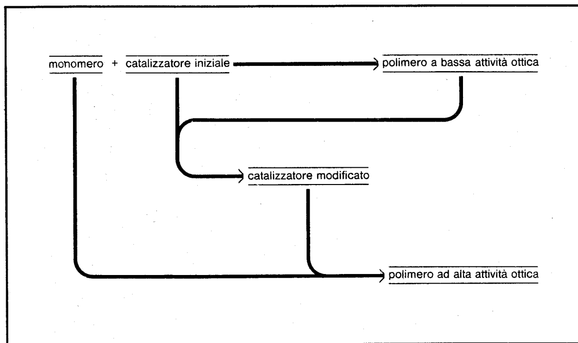
Fig.120 Schema della probabile azione del polimero sul processo di polimerizzazione asimmetrica. Mentre il catalizzatore iniziale ha un mediocre potere di induzione, il catalizzatore modificato dal polimero già formatosi è capace di indurre delle forti asimmetrie.
