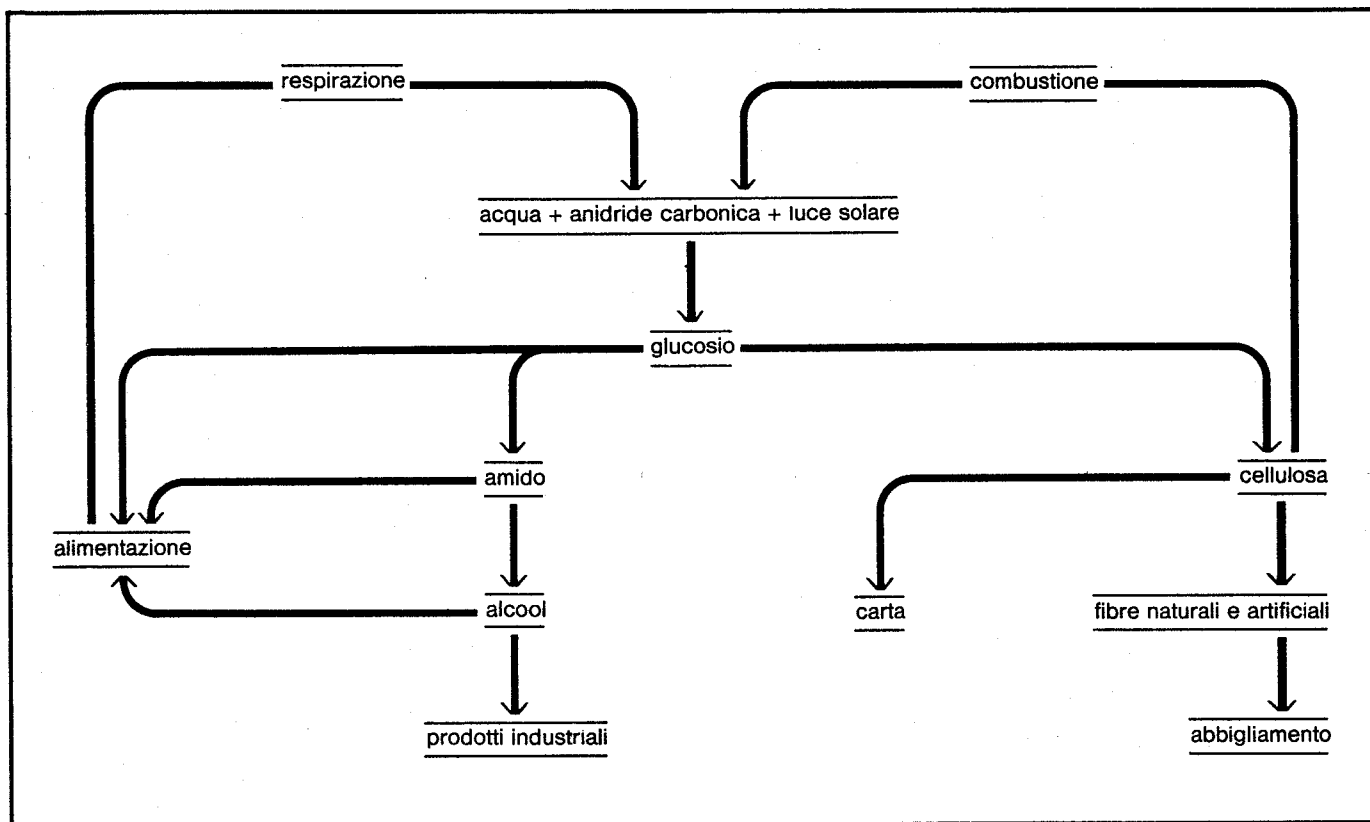
Fig.7 Rappresentazione schematica del ciclo di produzione e utilizzazione del glucosio.
