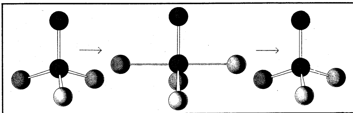
Fig.65 La reazione di sostituzione AX + Y^- = AY + X viene invece chiamata S_N2 quando segue una cinetica del secondo ordine ( v = K[A][B] ). La specie attivata è costituita da un complesso (YAX)^- a forma di bipyramide trigonale con l'agente nucleofilo e il gruppo uscente opposti fra loro. Il prodotto di reazione AY ha configurazione opposta a quella di AX perché il gruppo entrante si è avvicinato dalla parte opposta rispetto a X.
