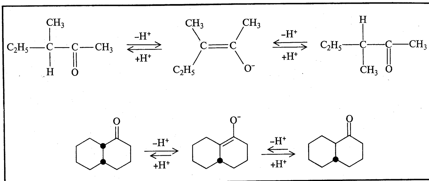
Fig.73. Il sec -butilmetilchetone otticamente attivo racemizza rapidamente in ambiente alcalino. L'intermedio di reazione indicato al centro contiene un piano di simmetria e si converte con ugual probabilità nel composto D e in quello L. Viceversa un chetone con due atomi di carbonio asimmetrico come il cis - \alpha -decalone si trasforma nell'isomero trans piú stabile, ma non racemizza. Uno degli atomi asimmetrici non viene toccato in questa reazione. Contrariamente al caso precedente l'intermedio di reazione è asimmetrico.
