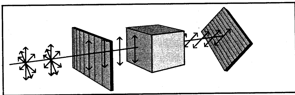
Fig.3 Se un raggio di luce polarizzata attraversa una sostanza otticamente attiva, il piano di polarizzazione si sposta dalla posizione iniziale ruotando di un angolo definito. La misura dell'angolo di rotazione viene ottenuta mediante un secondo polarizzatore: la posizione in cui si ha estinzione del raggio è infatti spostata rispetto ad una misura di confronto fatta in assenza del composto attivo. Coi moderni polarimetri fotoelettrici si possono misurare gli angoli con la precisione di un decimillesimo di grado. Il valore dell'attività ottica (o potere rotatorio) viene espresso come attività specifica [\alpha] = \alpha/d \cdot l , dove d è la densità del composto (se è un liquido puro) o la sua concentrazione (se è una soluzione) espressa in \text{g/cm}^3 e l è la lunghezza del tubo polarimetrico espressa in decimetri. Il potere rotatorio varia con la temperatura e con la lunghezza d'onda della luce usata; per questo si usa una luce monocromatica, generalmente la riga D emessa dal sodio. In modo più accurato si può misurare l'attività ottica a diversa lunghezza d'onda e tracciare la curva di dispersione rotatoria (variazione di [\alpha] in funzione di \lambda , lunghezza d'onda).
