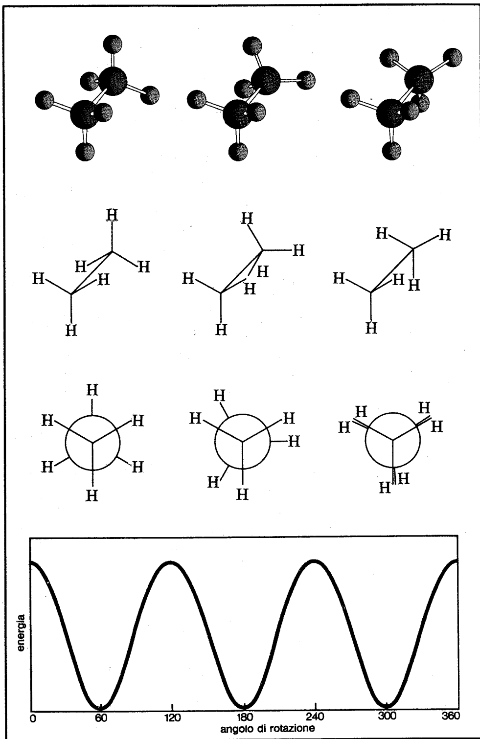
Fig.34 Modello molecolare, formula prospettica e proiezione di Newman di tre conformeri della molecola dell'etano \text{CH}_3\text{—CH}_3 . Le proiezioni di Newman si ottengono guardando la molecola lungo il legame attorno al quale avviene la rotazione. Si indica con un cerchio l'atomo inferiore e con un punto quello superiore. Le tre valenze residue si dispongono a 120^\circ fra loro. A sinistra conformazione sfalsata o staggered (con angoli di rotazione di 60^\circ , 180^\circ o 300^\circ ), al centro conformazione generica, a destra conformazione eclissata o eclipsed (con angoli di rotazione di 120^\circ , 240^\circ o 360^\circ ). In basso, profilo dell'energia potenziale della molecola in funzione dell'angolo di rotazione. I minimi di energia sono posti a 60^\circ , 180^\circ , 300^\circ , corrispondenti alle conformazioni sfalsate che risultano quindi le più stabili. L'altezza delle barriere di potenziale è di circa 3000 calorie per mole.
