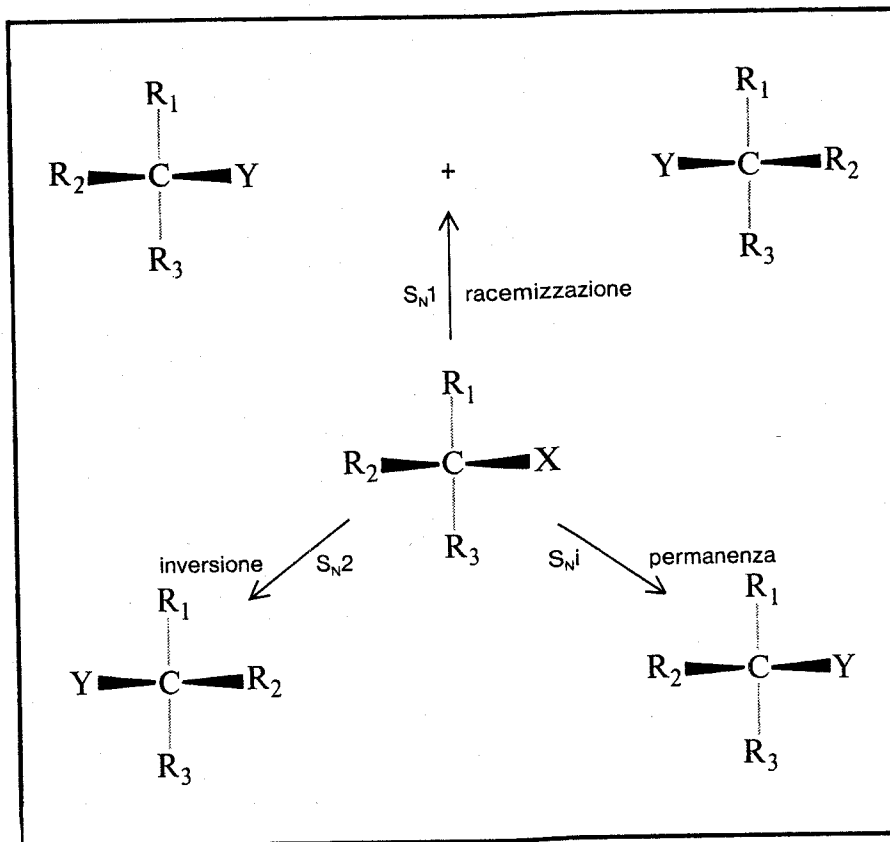
Fig.63 Decorso sterico delle reazioni S_N1 e S_N2 : esse danno luogo rispettivamente alla racemizzazione e all'inversione della configurazione. Altre reazioni di sostituzione meno comuni che avvengono con ritenzione di configurazione vengono chiamate S_{Ni} , sostituzioni nucleofile interne.
