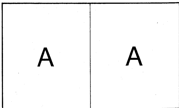
Fig.43 Il rettangolo in cui sono inscritte le lettere A è diviso in due parti speculari da una linea di riflessione: ogni punto a destra della linea è collegato con il suo simmetrico a sinistra da un'operazione di riflessione. Se si passa a una figura tridimensionale (si veda il cubo rappresentato a destra), l'operazione di riflessione deve essere riferita a un piano, detto piano di simmetria o piano speculare. Le due lettere incise sul dado sono in relazione fra loro come un oggetto e la sua immagine riflessa in uno specchio.
