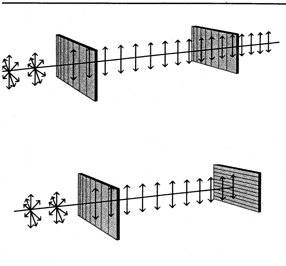
Fig.1 Quando un raggio luminoso passa attraverso un prisma di Nicol o una lamina Polaroid la luce viene polarizzata linearmente, possiede cioè un piano di vibrazione fisso ben definito. Un secondo polarizzatore parallelo al primo lascia passare la luce polarizzata; viceversa se viene orientato in modo perpendicolare provoca l'estinzione totale del raggio.
