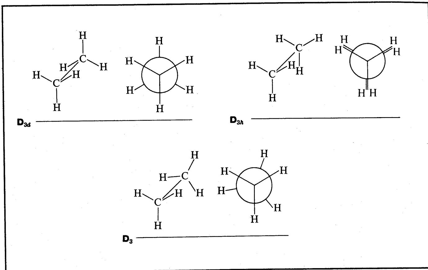
Fig.50 La conformazione stabile dell'etano possiede una simmetria D_{3d} ; in particolare essa possiede tre piani di simmetria che contengono ciascuno gli atomi di carbonio e due atomi di idrogeno. La conformazione eclissata, ad alta energia appartiene al gruppo D_{3h} e possiede anche un piano di simmetria che taglia il legame C—C. Le forme intermedie, pure instabili, hanno invece simmetria D_3 , hanno cioè assi di rotazione, ma non piani speculari: esse sono otticamente attive. Tuttavia, data la facilità di rotazione attorno al legame C—C, si può ritenere, a seconda dei casi, che la molecola dell'etano possieda la simmetria della sua forma stabile ( D_{3d} ) o anche una simmetria cilindrica ( D_{\infty d} ), come se fosse costituita da due sfere collegate a una bacchetta.
