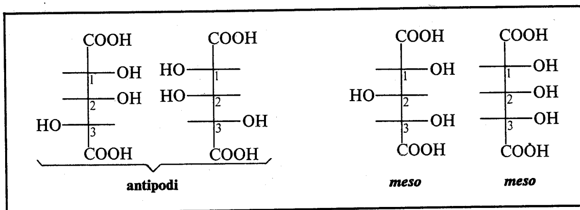
Fig.56 La proiezione di Fischer rappresenta una ipotetica conformazione non stabile della molecola: se essa contiene elementi di simmetria riflessiva, la molecola sarà costituita da conformazioni dissimmetriche antipode fra loro ed eventualmente da una o più conformazioni non-dissimmetriche. Se le barriere alla rotazione sono basse, le forme sono interconvertibili e il composto è inattivo ( meso ). Se invece la proiezione di Fischer è dissimmetrica, il composto è otticamente attivo: esistono perciò due antipodi configurazionali.
