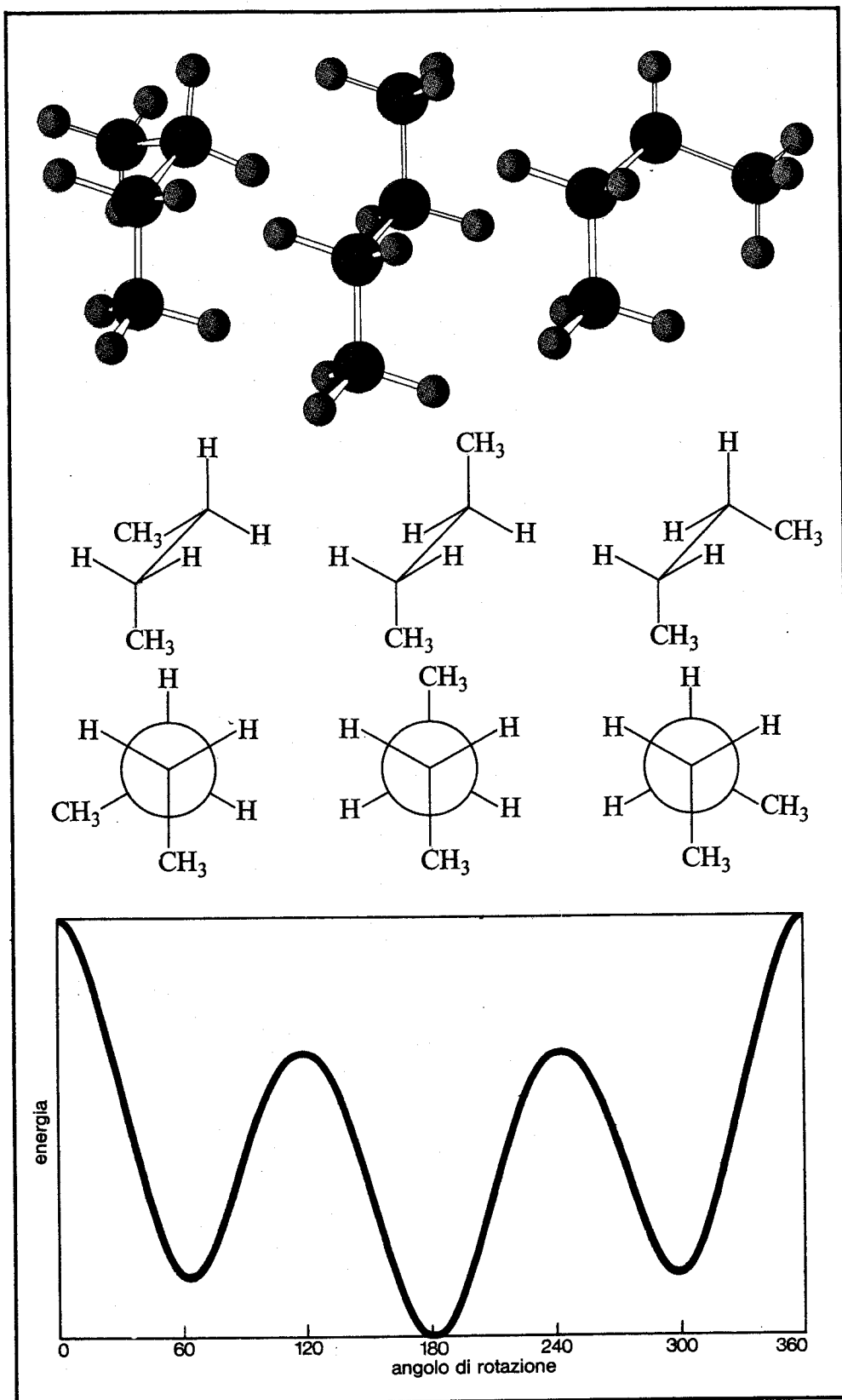
Fig.35 Modello molecolare, formula prospettica, e proiezione di Newman dei tre conformeri sfalsati del normal -butano C_4H_{10} : a sinistra una forma sghemba a 60^\circ (detta anche gauche o skew ), la forma anti (o trans , a 180^\circ ) e una seconda forma sghemba (a 300^\circ ), immagine speculare non sovrapponibile della prima. La forma più stabile, come si rileva dal profilo energetico, è quella anti , ma anche le forme sghembe hanno una reale esistenza (circa il 30% a temperatura ambiente) e la loro presenza è ancor più sensibile ad alta temperatura.
