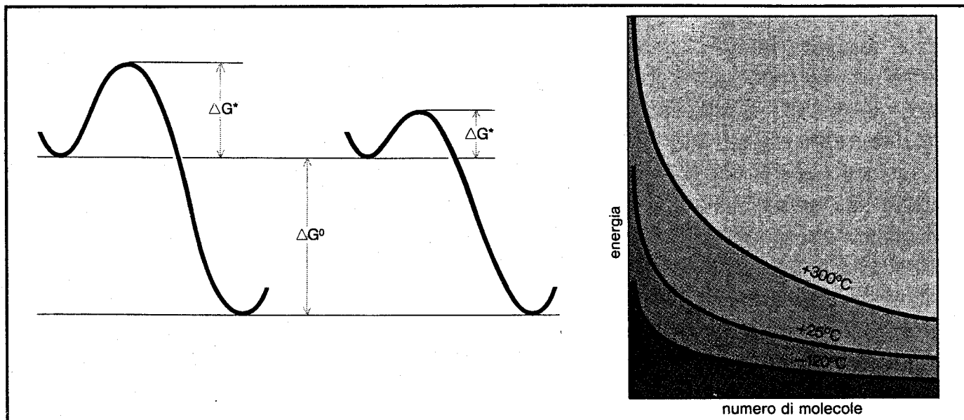
Fig.60 Una reazione chimica può avvenire solo se l'energia libera dello stato finale è inferiore a quella iniziale. A questa legge termodinamica si oppongono talvolta delle considerazioni cinetiche (relative alla velocità di reazione). Se l'energia di attivazione è alta, la reazione procede lentamente; se però si può ridurre l'altezza della barriera (ad esempio impiegando un catalizzatore), la velocità cresce anche di molti ordini di grandezza. Anche l'aumento della temperatura è generalmente favorevole ad un rapido corso della reazione: ad alta temperatura è infatti maggiore il numero di molecole dotate di energia sufficiente per superare la barriera energetica, come si può osservare nel diagramma a destra.
