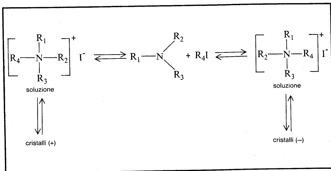
Fig.116 Le ammine terziarie reagiscono con gli ioduri alchilici per dare i sali di ammonio quaternario. Se i quattro gruppi alchilici legati all'azoto sono diversi fra loro si ha un fenomeno di enantiomorfismo analogo a quello che esiste nei composti del carbonio. Nel caso esaminato da Havinga i due antipodi si trasformano facilmente in soluzione l'uno nell'altro, ma cristallizzano nelle forme otticamente pure. La soluzione racema si può convertire nell'uno o nell'altro antipodo a seconda delle condizioni di cristallizzazione.
