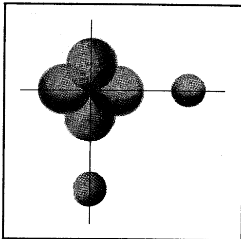
Fig.21 Combinazione di due orbitali 3p dello zolfo e dell'orbitale 1s di due atomi di idrogeno. Gli orbitali p sono ortogonali fra loro; ne deriva che anche l'angolo fra i legami nell'idrogeno solforato H_2S deve essere prossimo a 90^\circ .
