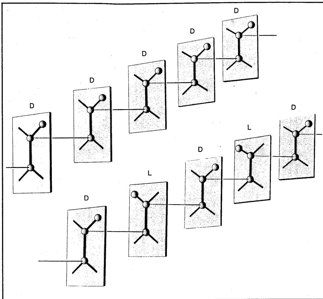
Fig.90 La stereochimica della polimerizzazione può essere spiegata introducendo due parametri: il tipo di addizione sul doppio legame ( cis o trans ) e il modo di presentazione del monomero alla catena crescente. Il propilene e gli altri monomeri vinilici sono prochirali, possono essere divisi in due parti enantiomorfe fra loro. Se il monomero reagisce sempre con la stessa faccia il polimero risulta isotattico, se reagisce alternatamente con le due facce risulta sindiotattico. Nella figura è indicato a titolo di esempio un tipo di addizione trans .
