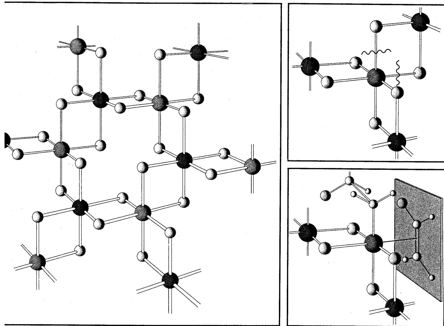
Fig.91 Frammento della cella cristallina del tricloruro di titanio di tipo \alpha . La struttura è localmente dissimmetrica, con alternanza di atomi di segno opposto (indicati con palline più chiare e più scure). L'altissima regolarità sterica del polipropilene isotattico potrebbe derivare dal fatto che ciascuna catena cresce su un atomo di titanio di un certo segno configurazionale e che il monomero si coordina a tale atomo sempre con la stessa faccia.
