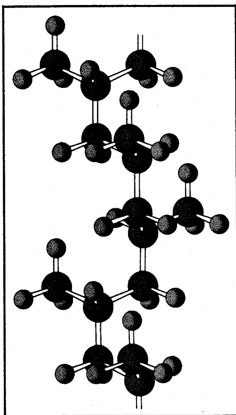
Fig.85 Conformazione ad elica ternaria del polipropilene isotattico allo stato cristallino. Gli angoli di rotazione interna sono alternatamente di 180^\circ e 60^\circ ; la catena può essere descritta come una successione di conformazioni T, G, T, G , ecc. ( T = trans o anti , G = gauche o sghemba ). I gruppi metilici sono disposti all'esterno in modo da rendere minima l'interazione col resto della catena.
