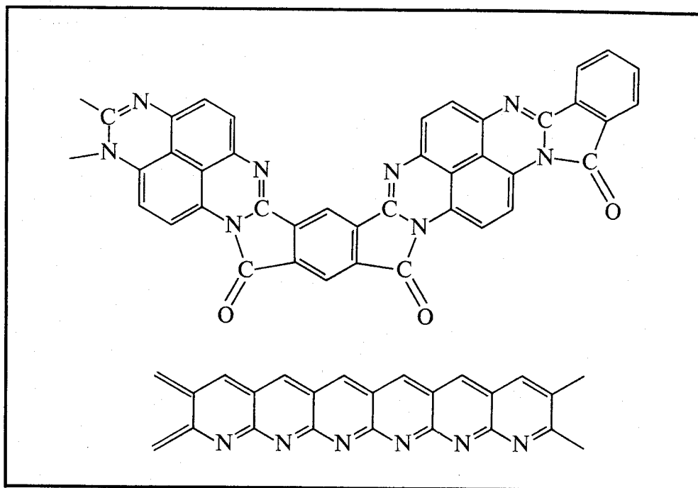
Fig.107 Due polimeri resistenti ad alta temperatura. Il primo è ottenuto per policondensazione di una tetrammina con un acido tetracarbossilico, il secondo per ciclizzazione e aromatizzazione di un polimero già formato, il poliacrilonitrile. Ambedue hanno una struttura policiclica rigida. La loro temperatura di fusione supera largamente i 400 °C.
