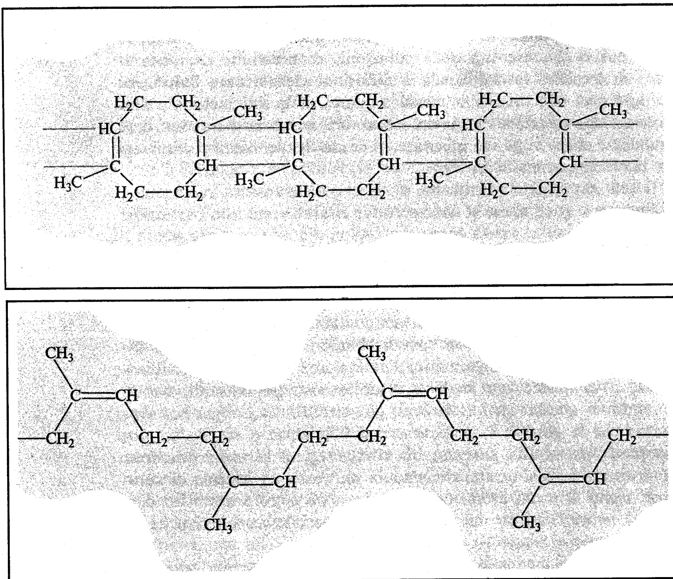
Fig.78 La struttura della gomma naturale, come viene interpretata oggi (in alto) e come era intesa cinquant'anni fa. Prima che la teoria macromolecolare fosse accettata si pensava all'esistenza di forze intermolecolari speciali le quali tenevano legate delle unità cicliche di basso peso molecolare e impartivano alla gomma le sue caratteristiche proprietà.
