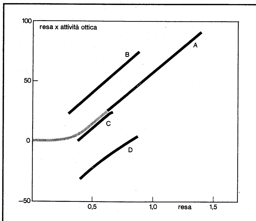
Fig.119 Un fenomeno di autocatalisi nella polimerizzazione del benzofurano. All'inizio della polimerizzazione l'attività ottica del polimero è molto bassa e raggiunge dei valori notevoli solo dopo che è stata ottenuta una certa quantità di polimero. Gli esperimenti compiuti in presenza di polimero preformato confermano l'ipotesi di una modifica del processo di polimerizzazione ad opera del polimero stesso. Nel diagramma in ascissa è riportata la resa di polimero, in ordinata il prodotto (resa di polimero \times potere rotatorio). Il valore dell'attività ottica del polimero è proporzionale all'inclinazione della curva. Il parallelismo tra le linee indica che il polimero che si forma ha il medesimo potere rotatorio in tutti i casi, indipendentemente dal segno ottico del polimero introdotto all'inizio.
