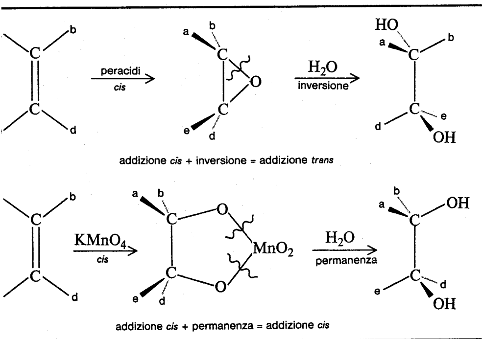
Fig.69 Talvolta il risultato finale di una reazione non coincide con quello del primo stadio. In alto, si ha dapprima un'addizione cis dell'ossigeno al doppio legame con formazione di un epossido; l'addizione di acqua avviene con inversione di configurazione e il risultato finale è trans . In basso, il passaggio dal composto ciclico a cinque atomi al glicol non coinvolge i legami carbonio-ossigeno e non altera quindi la configurazione.
