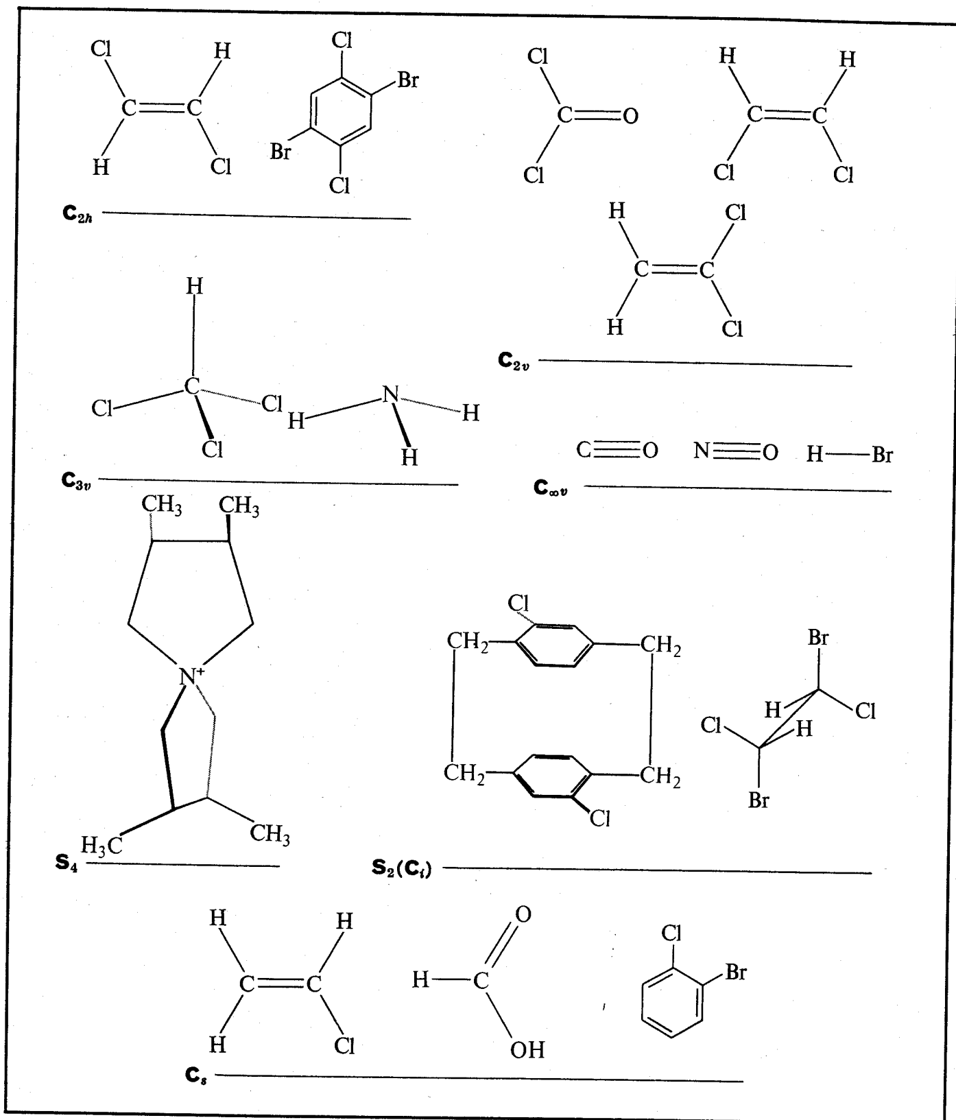
Fig.49 Esempi di molecole non dissimetriche. Al gruppo ottaedrico ( O_h ) appartengono il cromoesacarbonile e il cubano; al gruppo tetraedrico ( T_d ), il metano, l'adamantano, il nicheltetracarbonile; al gruppo D_{2d} , l'allene e il cicloottatetraene; al D_{3d} , il cicloesano; al D_{2h} , l'antracene; al D_{3h} , il trifluoruro di boro e il trifenilene; al D_{6h} , il benzene; al D_{\infty h} (simmetria cilindrica), l'acetilene, l'anidride carbonica e l'azoto. Esempi di altri gruppi sono i seguenti: gruppo C_{2h} , 1,4-dicloro,2,5-dibromobenzene, trans -dicloroetilene; gruppo C_{2v} , fosgene, cis -dicloroetilene, cloruro di vinilidene; gruppo C_{3v} , ammoniaca, cloruro di metile; gruppo C_{\infty v} (simmetria conica), l'ossido di carbonio, l'ossido di azoto, l'acido cloridrico. Al gruppo S_4 appartiene una tetrametilspiropirrolidina; al gruppo C_i , un dicloroparaciclofano e una particolare conformazione dell'1,2-dicloro,1,2-dibromoetano; infine al gruppo C_s , il cloruro di vinile, l'acido formico, l' orto -clorobromobenzene.
