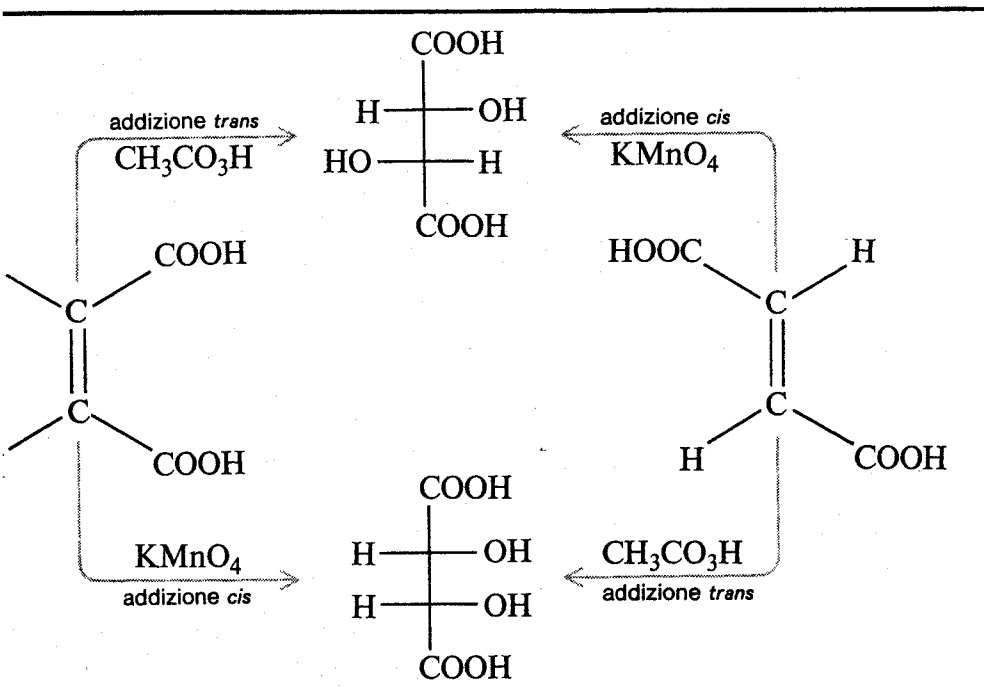
Fig.68 Per idrossilazione cis con permanganato ( \text{KMnO}_4 ) dall'acido maleico (a sinistra) si ottiene l'acido tartarico meso (in basso), mentre per idrossilazione trans con acido peracetico si ottiene l'acido tartarico racemo (in alto). Con gli stessi reagenti dall'acido fumarico (a destra) si ottengono rispettivamente l'acido racemo e l'acido meso -tartarico.
