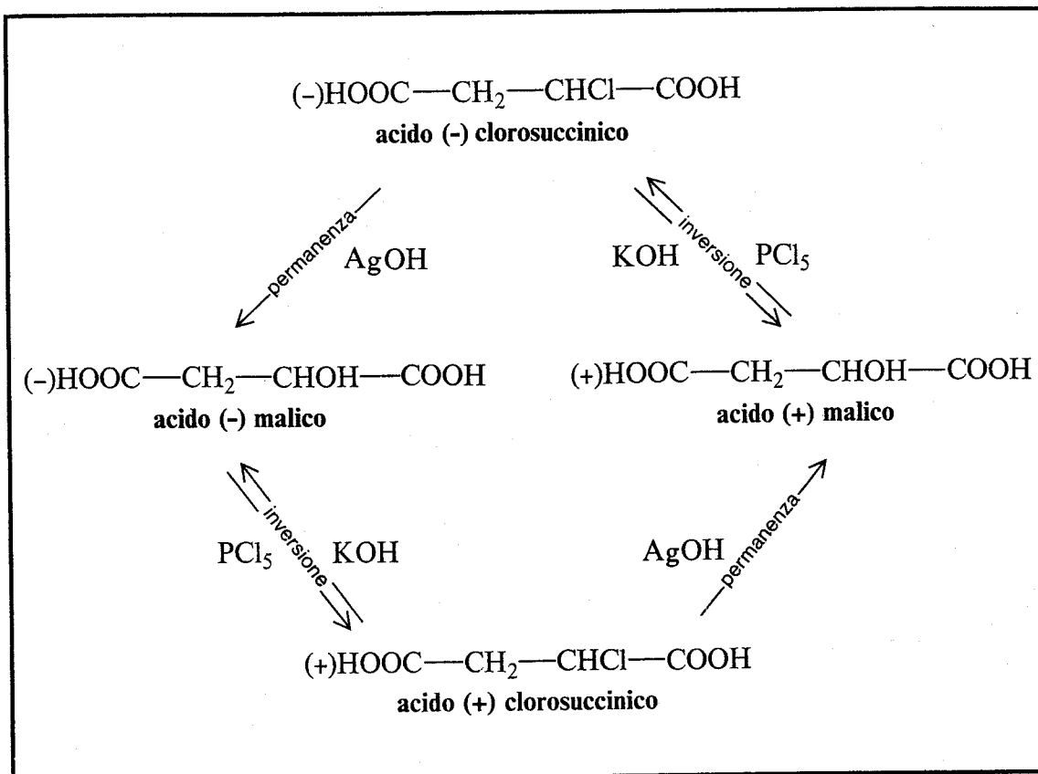
Fig.62 Nella conversione dell'acido malico nell'acido clorosuccinico e viceversa avvengono numerose inversioni di Walden o di configurazione. Le reazioni che si svolgono con ritenzione di configurazione sono assai piú rare di quelle che producono un'inversione.
