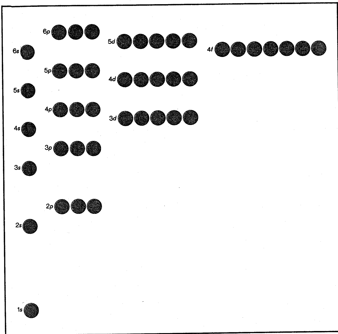
Fig.17 Rappresentazione dei livelli energetici approssimativi dei diversi orbitali atomici. Salendo dal basso si passa dall'orbitale più stabile (1s) agli orbitali più ricchi di energia. Il dislivello fra i differenti orbitali diminuisce man mano che l'energia aumenta.
