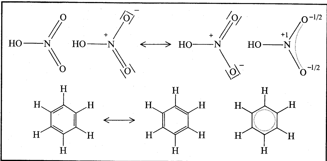
Fig.24 In alto, da sinistra: una formula ormai dimenticata dell'acido nitrico (in cui l'azoto è considerato pentavalente), due forme limite di risonanza che differiscono fra loro solo per la disposizione dei legami azoto-ossigeno, e formula con elettroni delocalizzati, intermedia rispetto alle forme limite. In basso, due forme limite di risonanza del benzene corrispondenti a quelle di Kekulé, e formula del benzene a simmetria esattamente esagonale.
