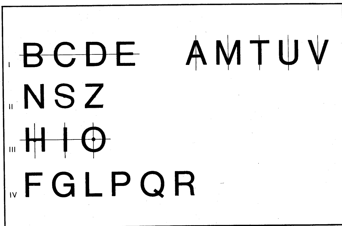
Fig.41 Le lettere maiuscole dell'alfabeto possono essere divise in quattro classi in base al tipo di simmetria. Nella prima, ciascuna lettera è divisa da una linea in due parti speculari; nella seconda, la rotazione di 180^\circ attorno a un asse verticale passante per il punto indicato lascia inalterata la forma della lettera; nella terza, questi due tipi di simmetria sono entrambi presenti; nella quarta, invece, non si nota alcun elemento di simmetria.
