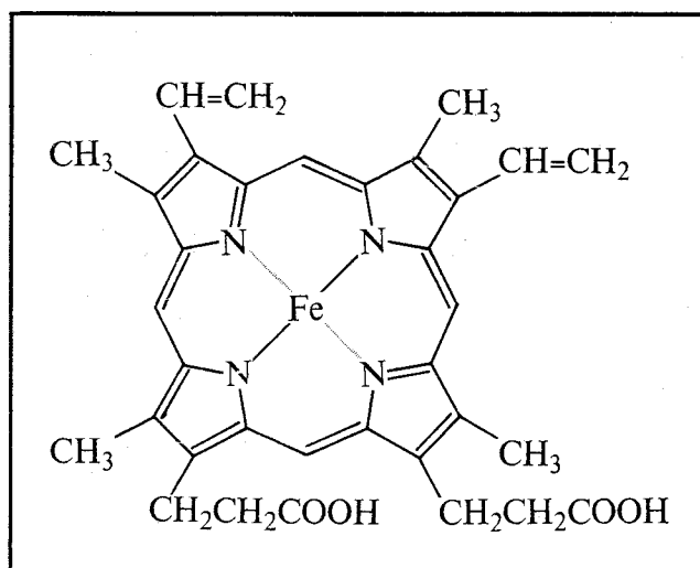
Fig.100 Struttura dell'emoglobina, come è stata determinata da Perutz: la risoluzione del dettaglio non è grandissima ma sufficiente per identificare la forma delle catene proteiche. A destra è riportata la formula chimica dell' eme , una molecola contenente un atomo di ferro e che è fissata all'interno delle anse della proteina.
