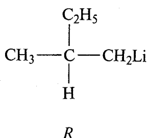
Fig.126 I due amminoacidi rappresentati in alto appartengono alla stessa serie sterica, ma il loro nome è opposto per la diversa priorità dei sostituenti. In basso: la reazione fra il cloruro di isoamile ( S ) e il litio non altera la configurazione dell'atomo asimmetrico, ma il nuovo composto ha configurazione R . L'ordine dei sostituenti è infatti il seguente: \text{CH}_2\text{Cl} > \text{C}_2\text{H}_5 > \text{CH}_2\text{Li} > \text{CH}_3 > \text{H} .
