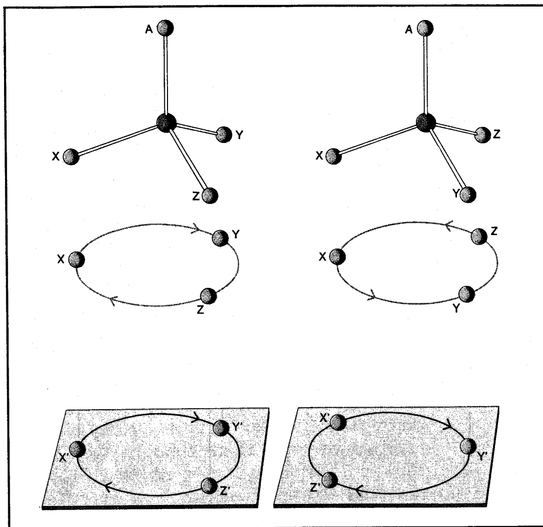
Fig.110 La teoria dei tre punti prevede che uno solo dei due antipodi si combini con un ricettore asimmetrico (a sinistra). L'altro antipodo avrà al massimo due punti di contatto. Pur essendo utile in alcuni casi particolari, questa teoria non ha validità generale.
