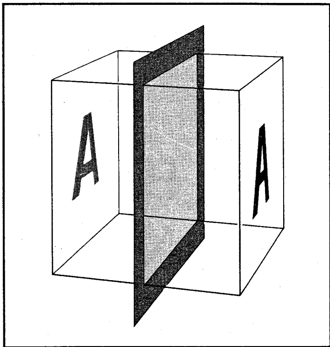
Fig.43 Il rettangolo in cui sono inscritte le lettere A è diviso in due parti speculari da una linea di riflessione: ogni punto a destra della linea è collegato con il suo simmetrico a sinistra da un'operazione di riflessione. Se si passa a una figura tridimensionale (si veda il cubo rappresentato a destra), l'operazione di riflessione deve essere riferita a un piano, detto piano di simmetria o piano speculare. Le due lettere incise sul dado sono in relazione fra loro come un oggetto e la sua immagine riflessa in uno specchio.
