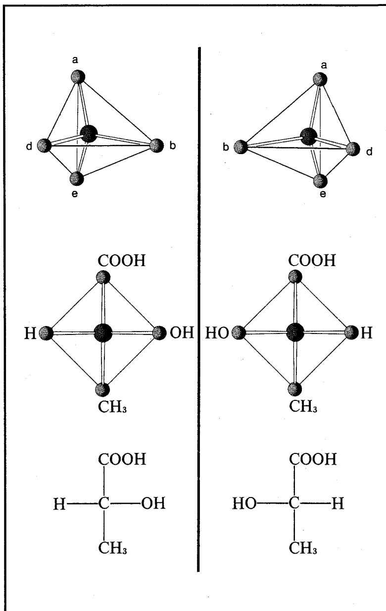
Fig.5 Solo una disposizione tetraedrica dei sostituenti permette l'esistenza di antipodi ottici in composti del tipo CABDE e la contemporanea assenza di isomeri in composti del tipo CAABB. La figura in alto a sinistra è l'immagine speculare non sovrapponibile di quella a destra. Ai fini di una rappresentazione convenzionale delle strutture tridimensionali, il tetraedro viene osservato dall'alto, dopo averlo appoggiato su uno spigolo in modo che lo spigolo superiore appaia orizzontale sul disegno (al centro). Eliminando i contorni del tetraedro si ottiene la proiezione di Fischer del composto, nel caso particolare l'acido lattico negativo (a sinistra) e positivo. In questa proiezione (in basso) le valenze verticali escono al di sotto del foglio, quelle orizzontali sono dirette verso l'alto.
