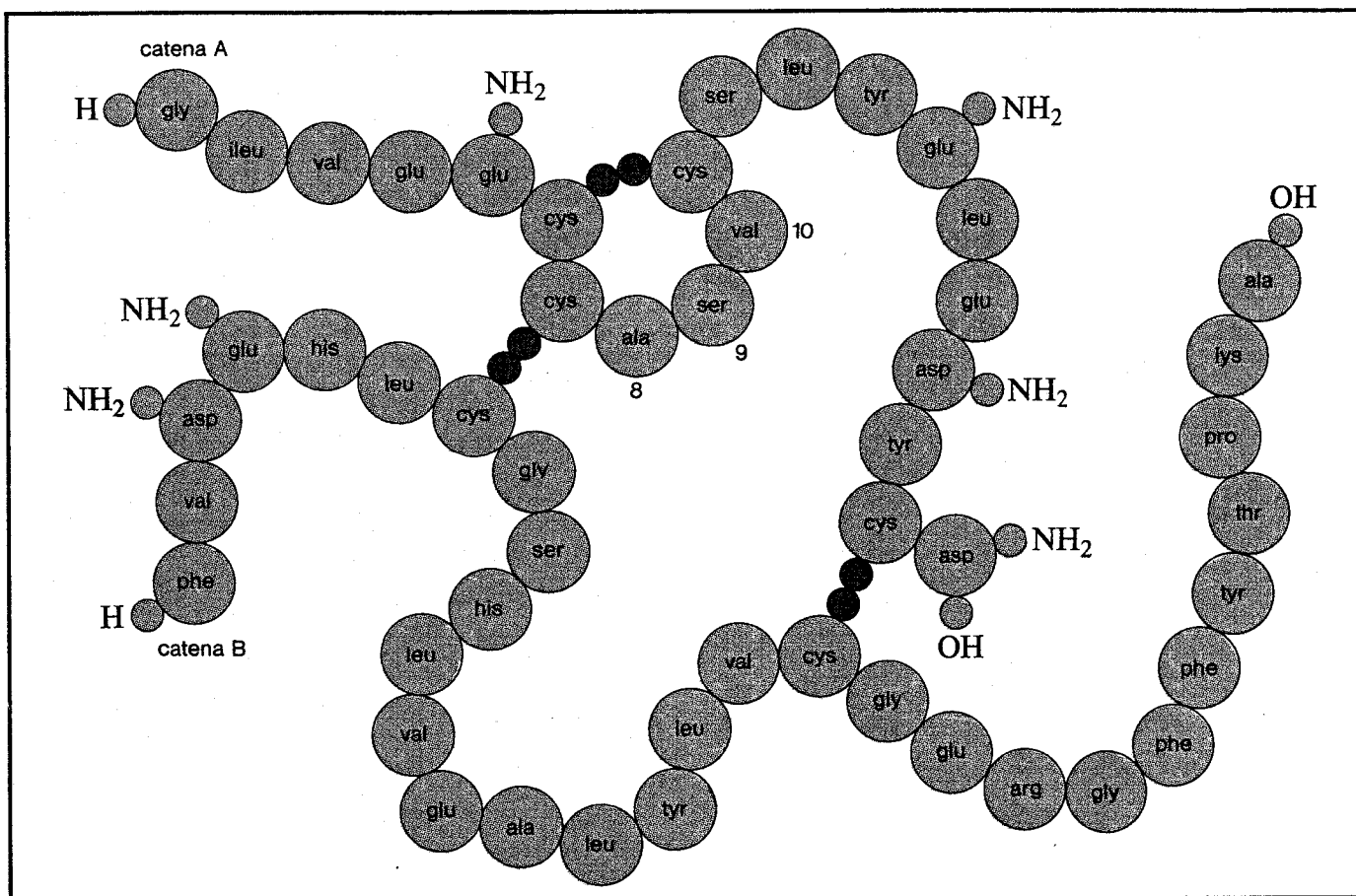
Fig.98 Rappresentazione convenzionale della molecola dell'insulina di bua. I cerchi grandi rappresentano i singoli amminoacidi, quelli piccoli chiari i gruppi laterali e terminali, quelli scuri i ponti a zolfo. L'insulina, formata da due catene peptidiche contenenti rispettivamente 21 e 30 amminoacidi, è stata recentemente sintetizzata da scienziati cinesi.
