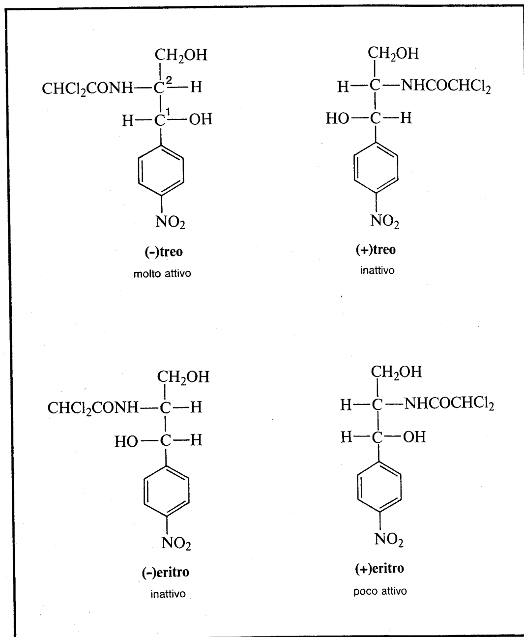
Fig.109 Solo uno dei quattro stereoisomeri del cloramfenicolo è molto attivo farmacologicamente, un altro ha un'azione assai ridotta e due sono inattivi. I due composti attivi hanno uguale configurazione sull'atomo asimmetrico 1, ma hanno segno ottico opposto.
