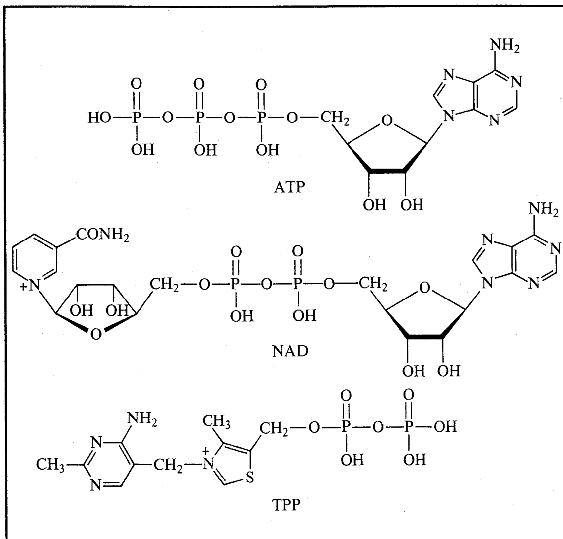
Fig.111 Formula di alcuni fra i più importanti coenzimi: da sinistra, l'adenosintrifosfato (ATP), il nicotinammidoadenindinucleotide (NAD) e il tiaminpirofosfato (TPP).
