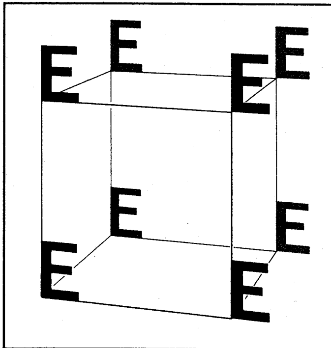
Fig.44 Tre esempi di simmetria per traslazione nelle figure in alto, in basso e a destra secondo una, due e tre dimensioni rispettivamente. Nel primo caso si ha una figura lineare; nel secondo, una figura piana; nel terzo, una figura solida o tridimensionale.
