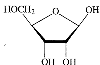
ribosio
