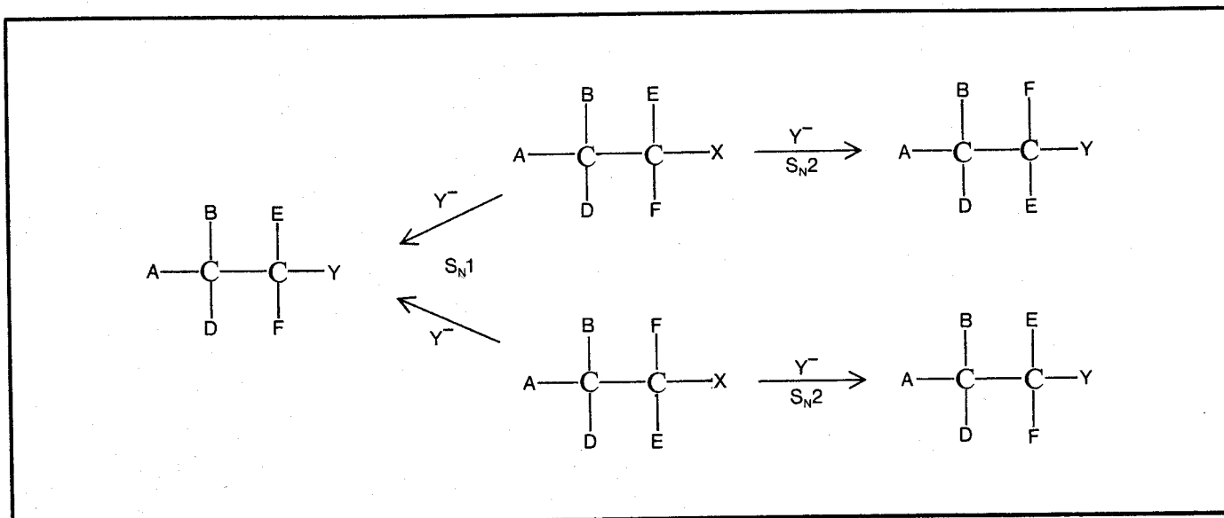
Fig.71 Una reazione di sostituzione del tipo S_N1 compiuta sui due diastereoisomeri di un composto con due atomi di carbonio asimmetrico conduce ad un unico prodotto (o ad una miscela in cui il componente maggiore è sempre lo stesso), quello termodinamicamente più stabile. Viceversa, se la reazione decorre con un meccanismo S_N2 , si ottengono due prodotti differenti. In quest'ultimo caso si ha un controllo sterico di tipo cinetico.
