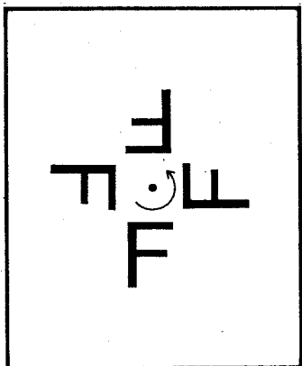
Fig.42 Un quadrato in cui siano inscritte nel modo indicato quattro lettere uguali rappresenta un esempio di simmetria rotazionale quaternaria: si dice che è presente un asse di simmetria del quarto ordine, la cui proiezione sul piano è indicata da un punto. A destra è rappresentato un cubo avente quattro facce contraddistinte da una lettera. Si ha anche qui un asse di rotazione del quarto ordine. Analogamente gli assi binari o ternari impongono un ricoprimento della figura due o tre volte per ogni rotazione completa.
