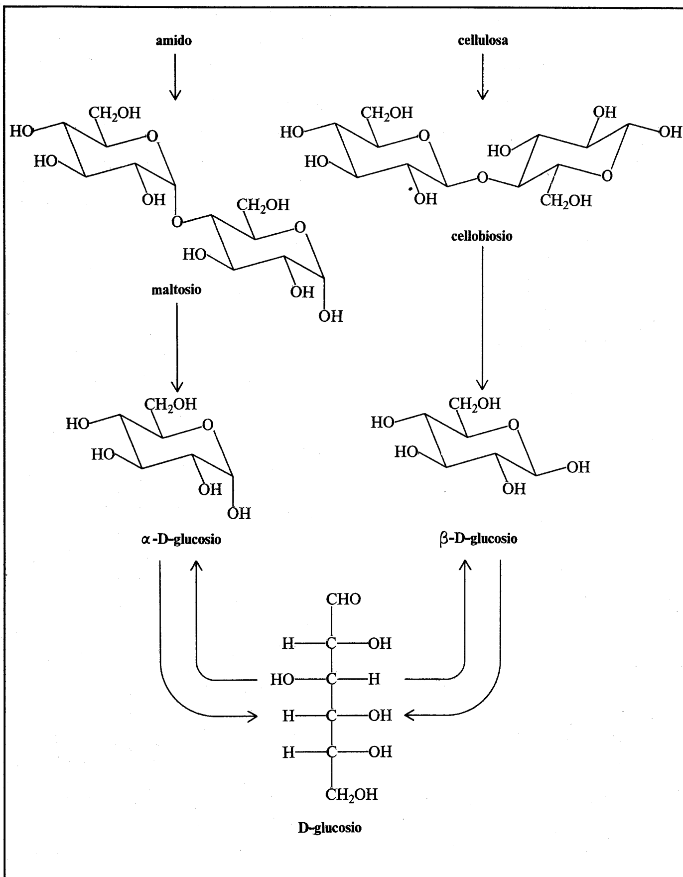
Fig.95 La degradazione dell'amido e delle cellulosa porta ad un medesimo prodotto, il D-glucosio, attraverso intermedi diversi. L'amido si trasforma in maltosio, un derivato dell' \alpha -glucosio, mentre la cellulosa si converte nel cellobiosio a sua volta formato da due unità di \beta -glucosio; \alpha - e \beta -glucosio sono facilmente convertibili in soluzione l'uno nell'altro.
