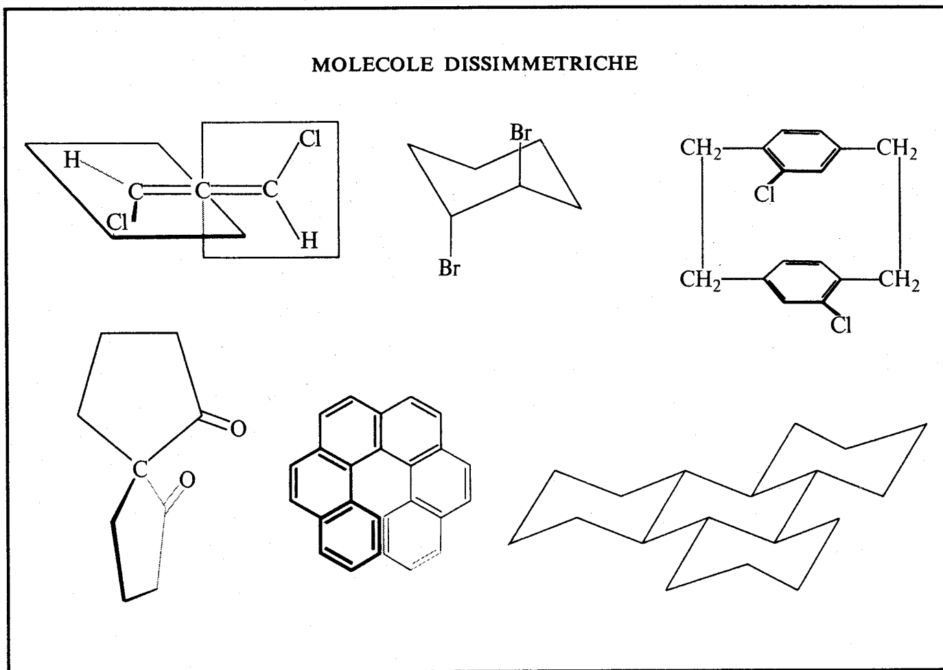
Fig.48 Le molecole dissimmetriche non hanno assi alternanti di simmetria, ma solo assi di rotazione semplice. In figura, alcuni composti del gruppo C_2 : il dicloroallene, l'1,2- trans -dibromocicloesano, un dicloroparaciclofano, un chetone spiranico e l'elicene. Al gruppo D_2 appartiene l'ultimo composto, uno dei dieci isomeri del peridotrifenilene, la molecola organica a più alta simmetria finora separata in antipodi ottici.
