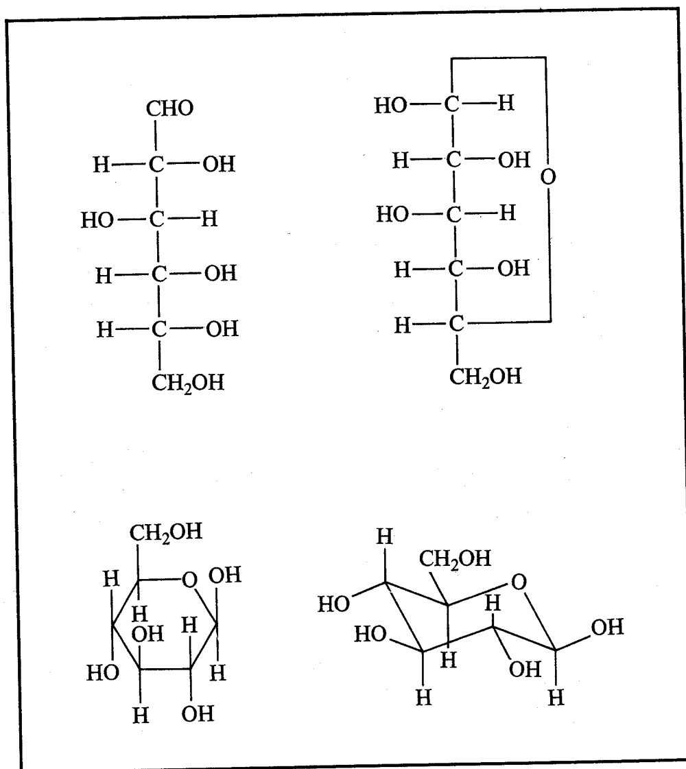
Fig.40 Dalla formula di Fischer del glucosio alla moderna rappresentazione della conformazione del \beta - glucopiranosio. In questo composto tutti i sostituenti sono equatoriali.
