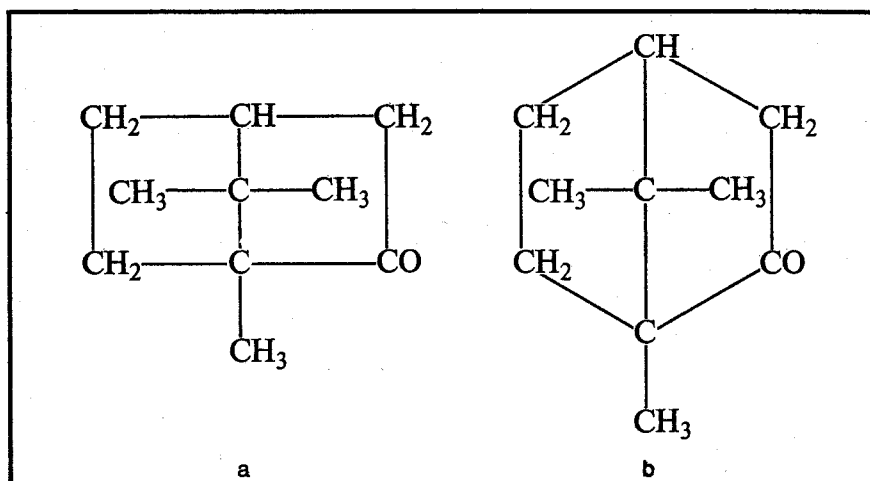
Fig.28 Le vecchie formule della canfora (in alto) danno un'idea poco corretta della sua reale struttura (c). La formula (d) ne è invece una trascrizione grafica abbastanza efficace, che mette in evidenza la non planarità dello scheletro molecolare e la possibilità di isomeria dei derivati della canfora.
