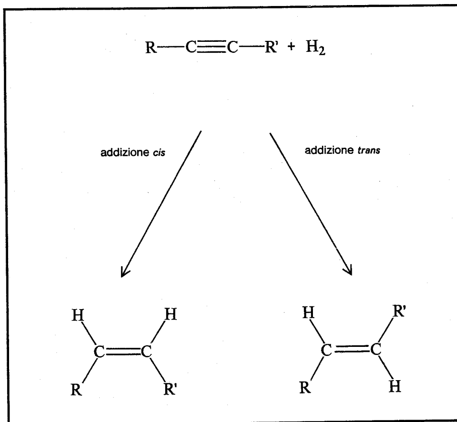
Fig.66 Un processo di addizione su un composto acetilenico viene detto di tipo cis (o trans ) quando i due atomi introdotti nella molecola si trovano in posizione cis (o trans ) rispetto al doppio legame.
