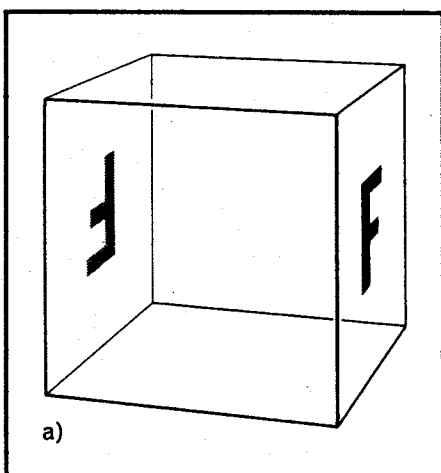
Fig.45 In a), esempio di figura con centro di simmetria o di inversione. Ogni punto della lettera incisa su una faccia del dado è collegato al suo simmetrico sull'altra faccia da linee rette passanti per il centro del dado. Questo punto è il centro di simmetria o di inversione. Un semplice esempio è rappresentato dall'obiettivo fotografico. La differenza tra centro di simmetria in a), piano di simmetria in b) e asse di rotazione binario in c) è chiaramente visibile dal confronto delle tre figure.
