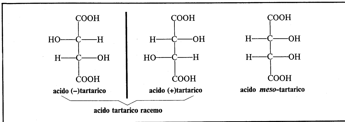
Fig.6 Formule in proiezione di Fischer. Da sinistra, l'acido tartarico negativo, quello positivo e l'acido mesotartarico. La configurazione dei due atomi asimmetrici è uguale nei primi due composti e opposta nel terzo.
