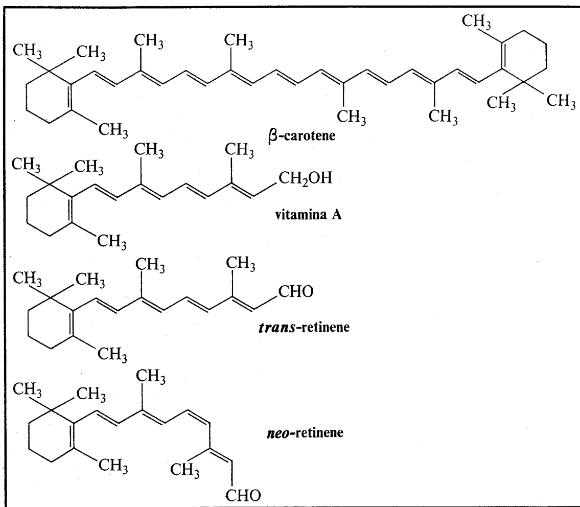
Fig.113 Formule di composti legati alla chimica della visione. Dall'alto, \beta -carotene, vitamina A, trans -retinene e neo -retinene. Gli ultimi due composti sono stereoisomeri del tipo cis-trans . L'alto grado di insaturazione di queste molecole fa sì che esse siano sensibili alle radiazioni elettromagnetiche a lunghezza d'onda compresa fra 4000 e 7000 Å.
