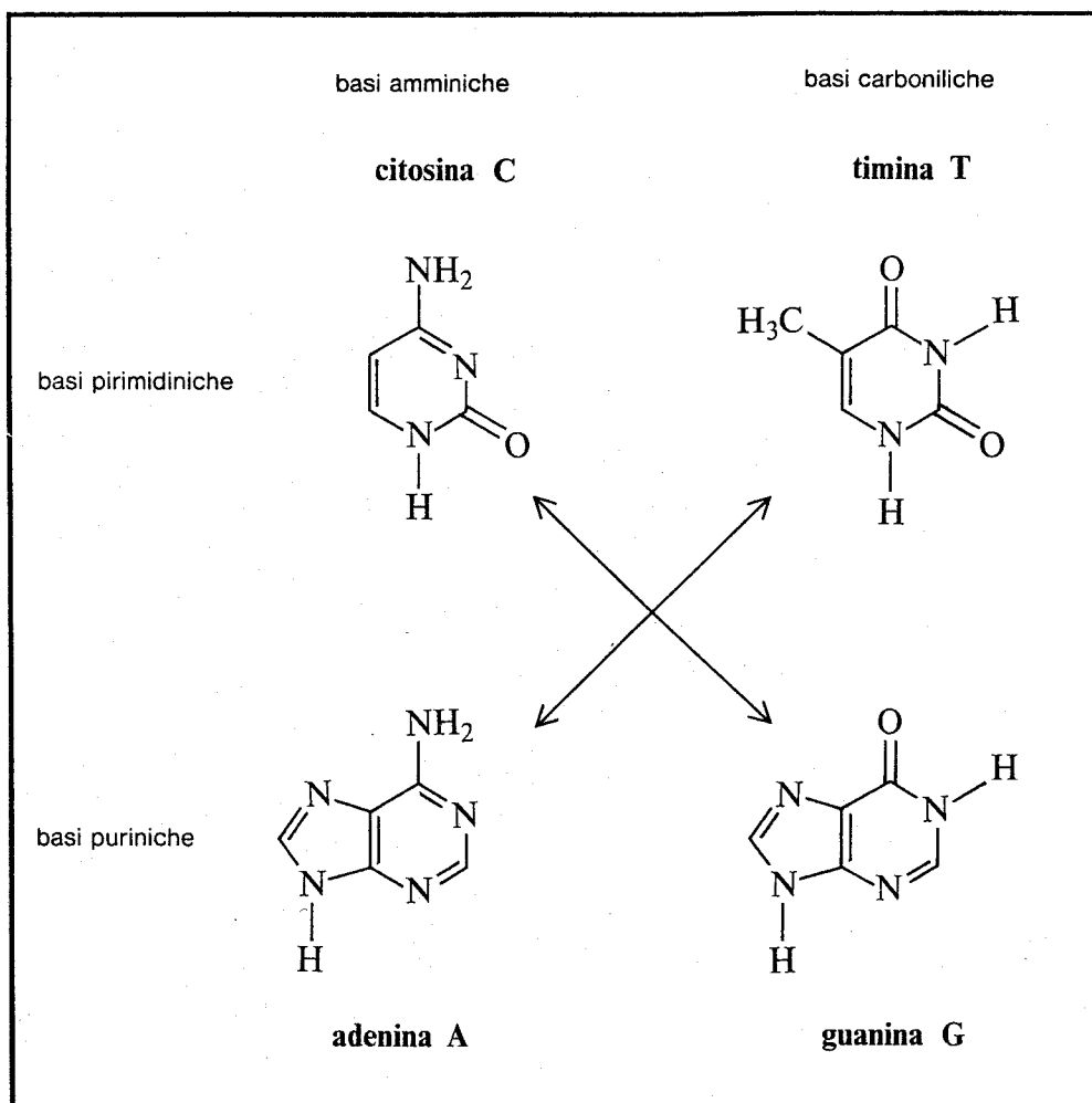
Fig.102 Le quattro basi del DNA. Le frecce indicano le coppie di basi complementari. Questa relazione, basata sull'analisi quantitativa e l'esame formale delle loro caratteristiche strutturali, ha un importante significato fisico.
