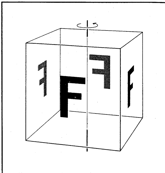
Fig.42 Un quadrato in cui siano inscritte nel modo indicato quattro lettere uguali rappresenta un esempio di simmetria rotazionale quaternaria: si dice che è presente un asse di simmetria del quarto ordine, la cui proiezione sul piano è indicata da un punto. A destra è rappresentato un cubo avente quattro facce contraddistinte da una lettera. Si ha anche qui un asse di rotazione del quarto ordine. Analogamente gli assi binari o ternari impongono un ricoprimento della figura due o tre volte per ogni rotazione completa.
