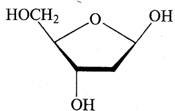
desossiribosio
