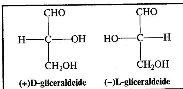
Fig.9 Proiezione di Fischer della formula della D- ed L-gliceraldeide. L'attribuzione della formula D al composto con rotazione ottica positiva è stata fatta da Fischer in modo puramente convenzionale. Tuttavia nel 1951 questa attribuzione è stata confermata sperimentalmente da Bijvoet mediante una esperienza di dispersione anomala dei raggi X (si veda anche a pag. 30).
