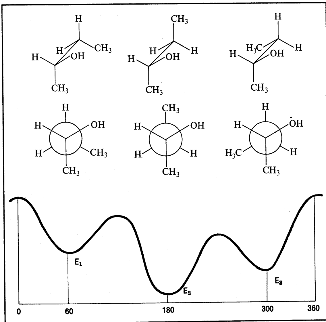
Fig.55 Le tre conformazioni stabili dell'alcool sec -butilico sono tutte dissimmetriche e non sono antipode tra loro: ciò dipende dalla presenza di un atomo di carbonio asimmetrico. L'energia delle tre conformazioni è diversa e il diagramma energetico non è simmetrico.
