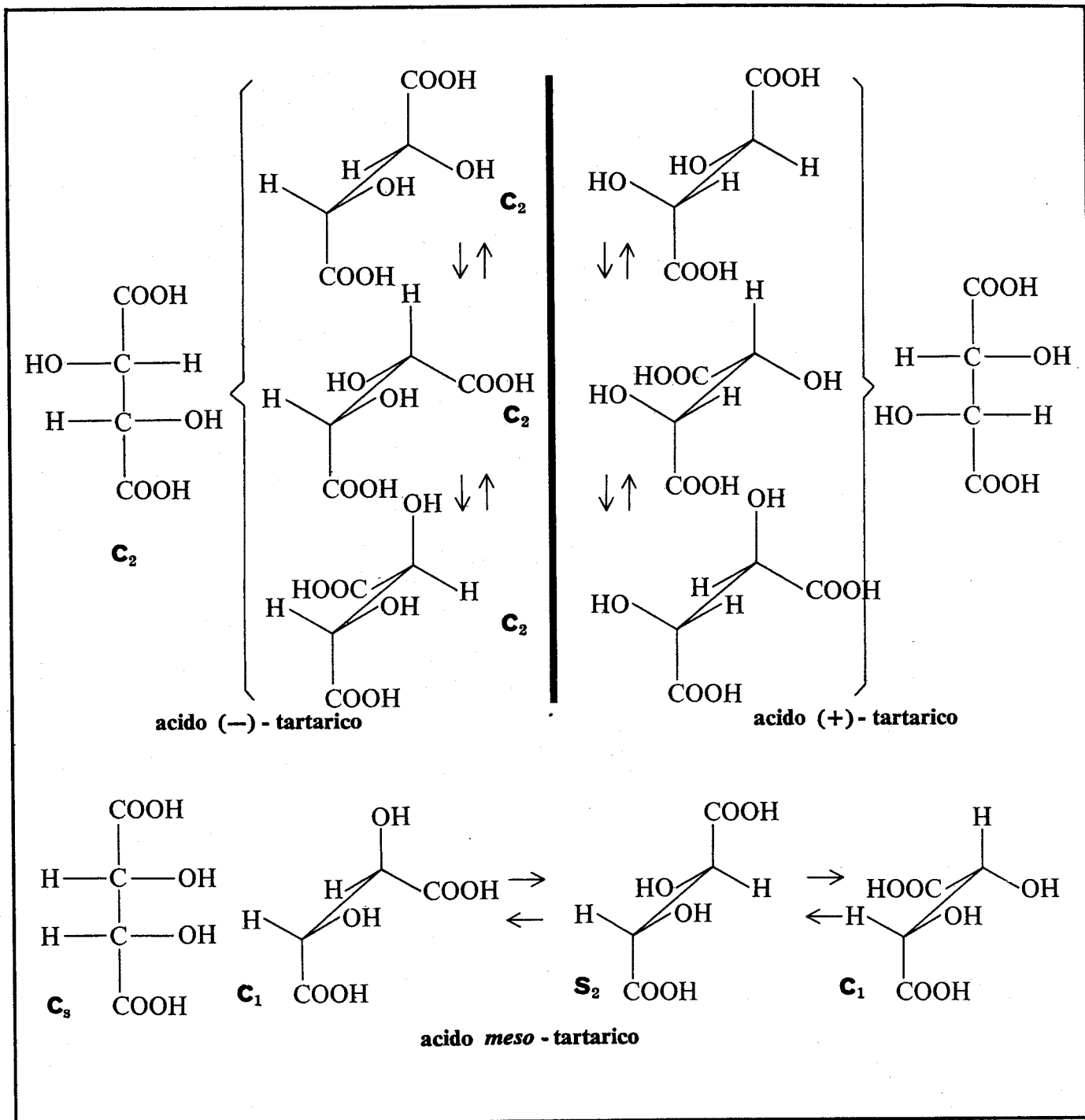
Fig.53 Proiezioni di Fischer e formule prospettiche degli acidi tartarici. In alto, a sinistra, l'acido (—)-tartarico: le conformazioni stabili sono tutte dissimmetriche ( C_2 ) e facilmente interconvertibili tra loro, ma non con le loro immagini speculari. Se costruiamo queste immagini speculari, otteniamo un altro composto, l'acido (+)-tartarico, che non può trasformarsi nel primo. Sotto: l'acido meso -tartarico (inattivo) può esistere in tre conformazioni interconvertibili, di cui una centrosimmetrica e le altre asimmetriche e antipode fra loro.
