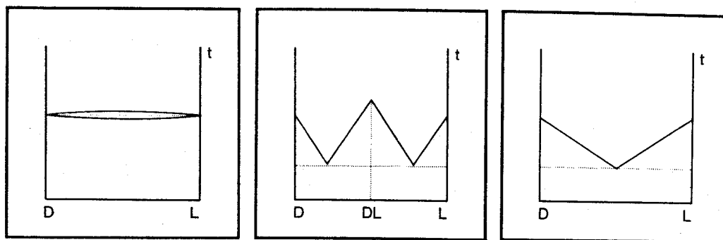
Fig.108. Diagramma di fusione delle miscele di antipodi. A sinistra, il punto di fusione è praticamente costante in tutto il campo di composizioni (si ha formazione di cristalli misti); al centro formazione di un racemato, i cui cristalli sono formati da ugual numero di molecole destre e sinistre; a destra formazione di una miscela eutettica bassofondente.
