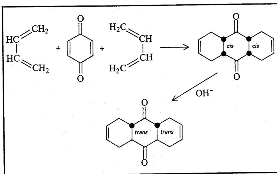
Fig.72 La reazione di Diels-Alder fra due molecole di butadiene e il benzochinone cis . Il chetone risultante può isomerizzare nell'isomero trans-trans più stabile mediante un trattamento con agenti alcalini.
