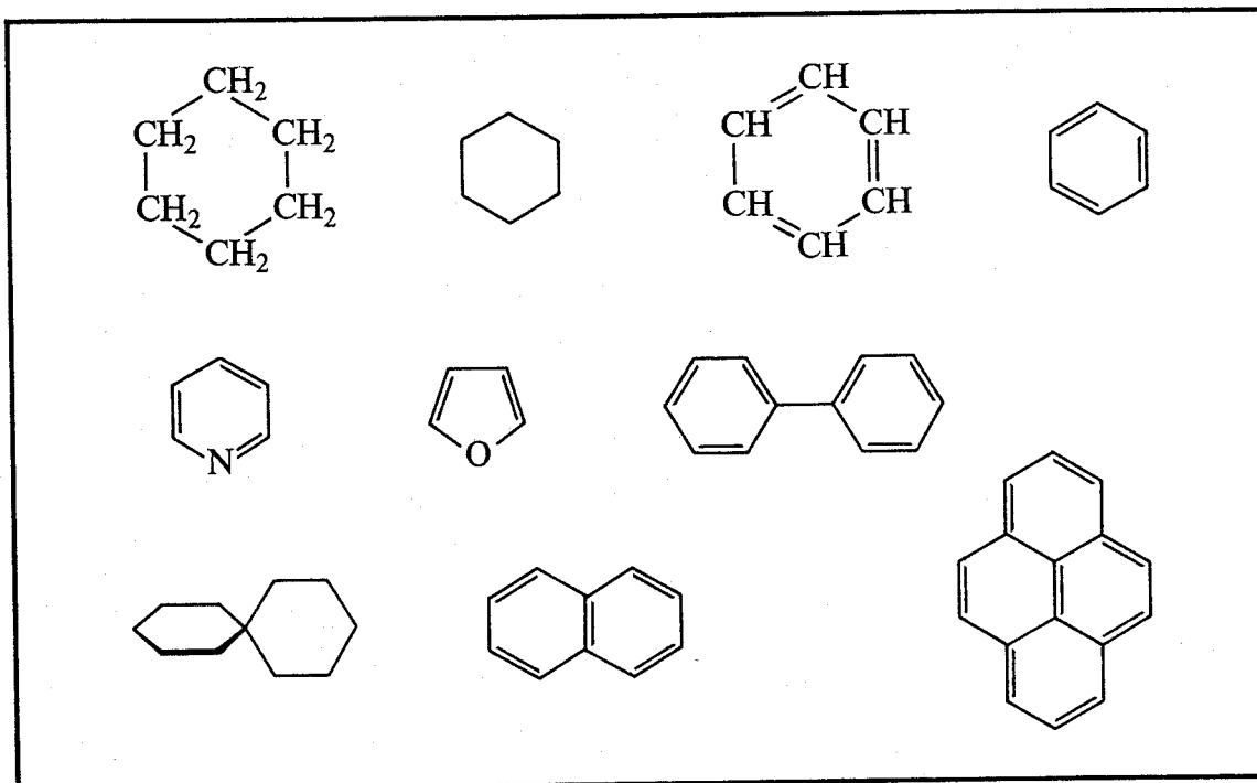
Fig.27 Formule di struttura di alcuni composti ciclici. Molto spesso nella rappresentazione grafica si omettono gli atomi di carbonio facenti parte dell'anello. Dall'alto e da sinistra sono riportate due formule del cicloesano e due del benzene, la formula della piridina e quella del furano; seguono le formule di alcuni composti policiclici: il difenile e lo spiro(5,5)undecano, detto anche cicloesanspirocicloesano, la naftalina e il pirene.
