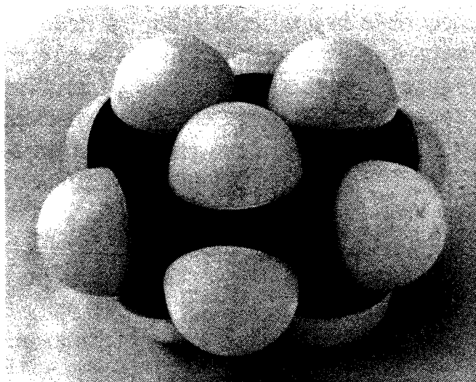
Fig.33 Tre diversi tipi di modelli molecolari. In alto è messo in evidenza lo scheletro della molecola: è ben visibile la posizione dei nuclei atomici, la lunghezza e l'angolo fra i legami e il dettaglio conformationale. In basso un modello a sfere, che dà un'idea dell'ingombro esterno della molecola. Il raggio delle sfere è uguale al raggio di Van der Waals dei diversi atomi, e corrisponde alla distanza alla quale si hanno delle forti azioni repulsive fra gli atomi vicini. Il modello corrisponde al cicloesano.
