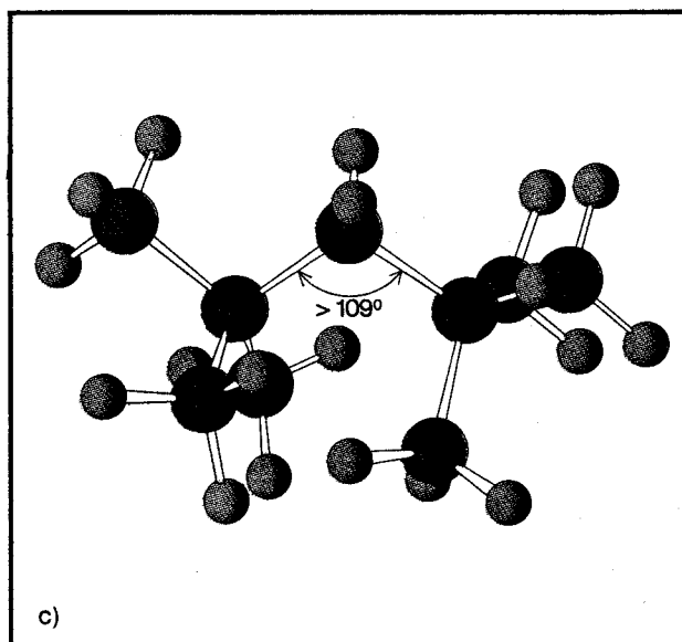
Fig.36 L'interazione fra atomi non direttamente legati, o interazione di Van der Waals, fra due gruppi metilici disposti come è indicato nella formula a1 dà alla molecola del 2,4-dimetilpentano un'energia troppo elevata. Per rotazione attorno ad un legame, la molecola si trasforma nella conformazione più stabile a2. Per il 2,2,4-trimetilpentano o iso -ottano non esiste alcuna conformazione sfalsata a bassa energia. La forma più stabile è quella con i due metili in basso eclissati rispetto ai due atomi di idrogeno centrali (b). Nel 2,2,4,4-tetrametilpentano la presenza di un ulteriore metile rende la molecola eccessivamente compressa: un'opportuna deformazione dell'angolo di valenza fa sì che i due atomi di carbonio quaternari si allontanino fra loro (c).
