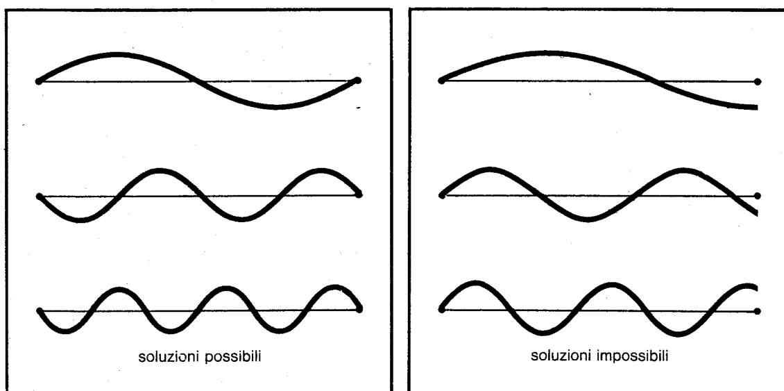
Fig.13 La lunghezza d'onda delle vibrazioni di una corda di violino è un sottomultiplo intero della lunghezza della corda (uno, un mezzo, un terzo, un quarto, ecc.). Tutte le altre frequenze di vibrazione sono impossibili perché non permettono l'esistenza di nodi agli estremi della corda. (I nodi sono i punti in cui l'ampiezza delle vibrazioni è nulla.)
