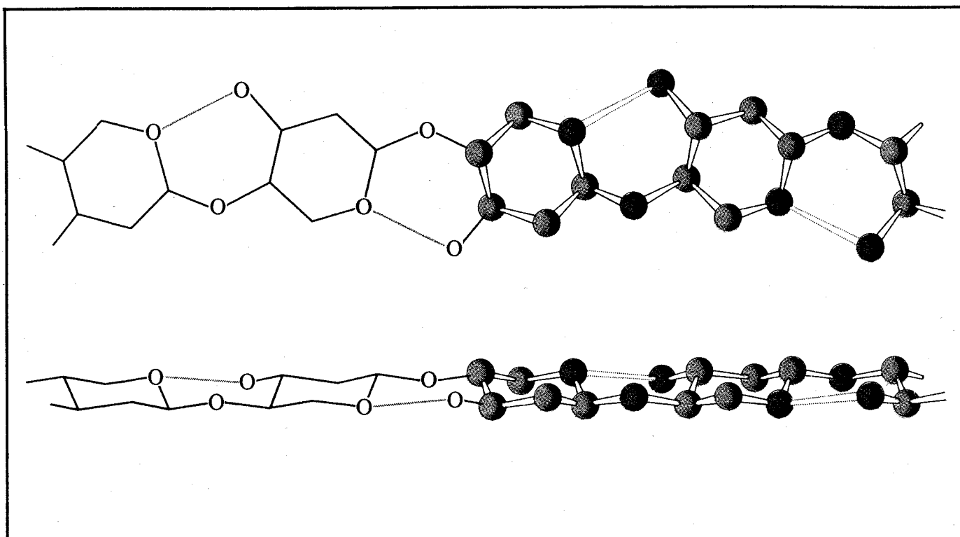
Fig.96 Una delle strutture proposte per la cellulosa: i legami a tratto nero sono covalenti, quelli più chiari sono legami a idrogeno fra atomi di ossigeno. Gli anelli glucosidici visti in piano nelle formule in alto esistono in realtà nella conformazione a sedia.
