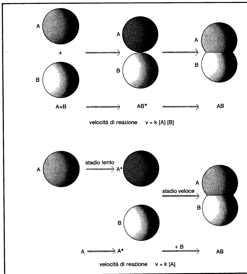
Fig.61 Illustrazione dei meccanismi bimolecolare e monomolecolare delle reazioni fra A e B. L'urto fra A e B porta alla formazione di un complesso attivato AB^* che si trasforma rapidamente nel composto AB (in alto). In basso: il reagente A si converte dapprima nella specie attivata A^* che successivamente reagisce con B per dare il prodotto finale.
