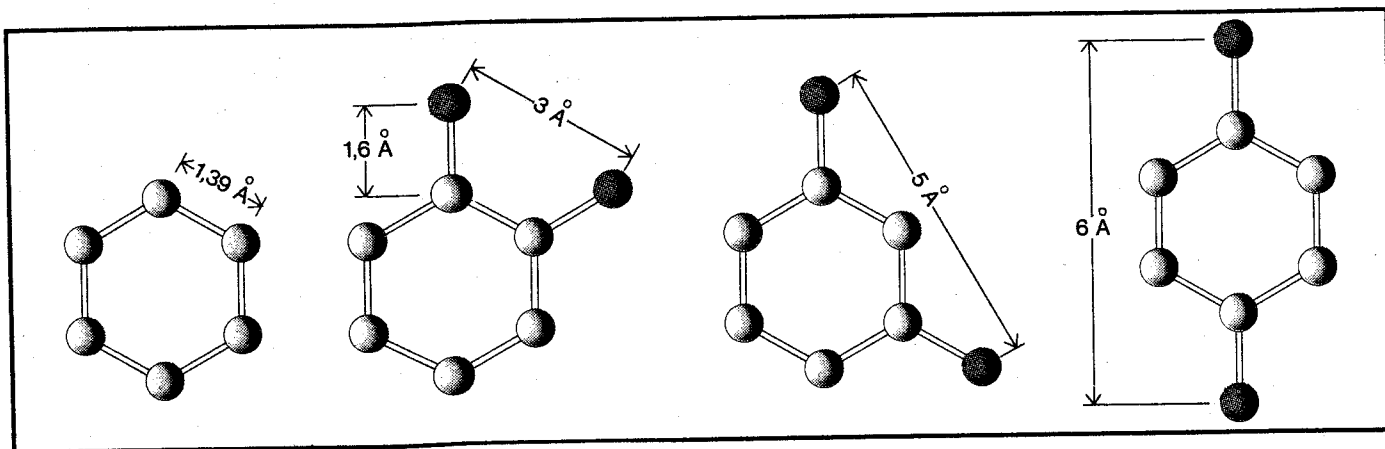
Fig.29 Modelli del benzene, dell'1,2 od orto -diclorobenzene, dell'1,3 o meta -diclorobenzene e dell'1,4 o para -diclorobenzene. Sono indicate le più significative distanze interatomiche tra gli atomi di carbonio nel benzene e tra gli atomi di cloro nei derivati clorurati.
