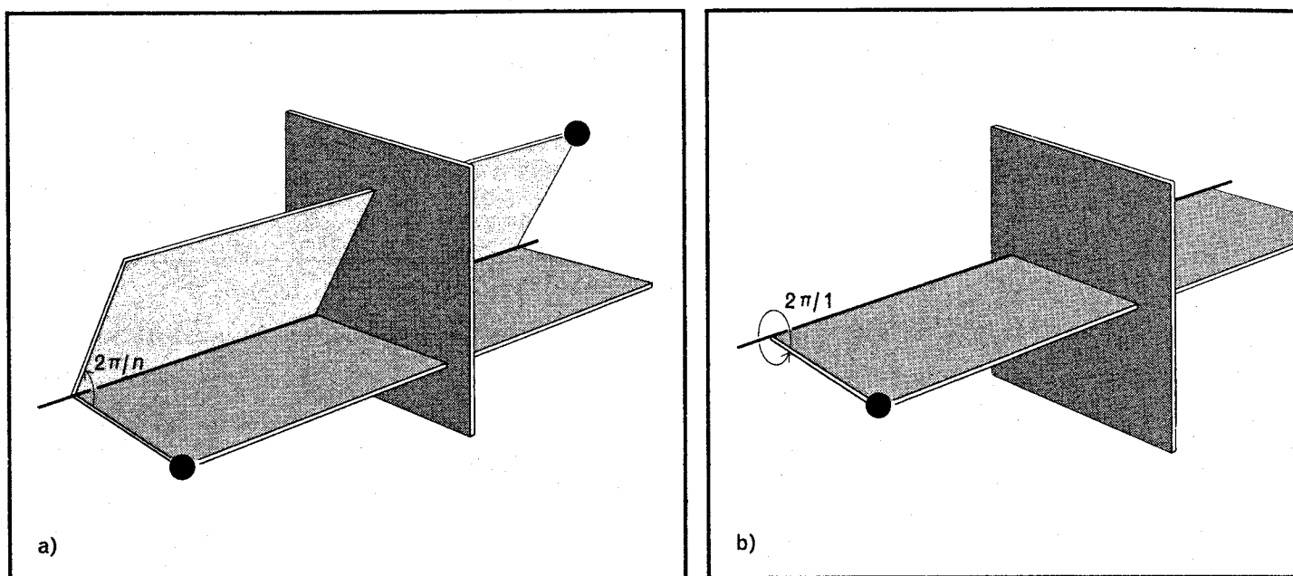
Fig.46 L'asse di rotoriflessione, detto anche asse alternante, è definito dalla combinazione di due operazioni di simmetria. Dapprima si compie una rotazione attorno all'asse di un certo angolo ( 2\pi/n , se n è l'ordine dell'asse) e successivamente si opera una riflessione su un piano perpendicolare all'asse, come è illustrato in a).
