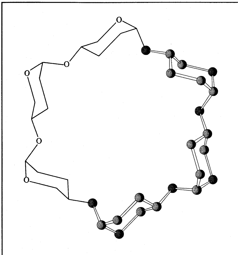
Fig.97 La ciclodestrina e l'amilosio sono strettamente apparentati sul piano chimico e strutturale. La prima è un composto ciclico a forma di ciambella contenente sei residui \alpha -glucosidici, il secondo è una macromolecola di forma elicoidale la cui proiezione su un piano è praticamente identica a quella della ciclodestrina. La sovrapposizione di molecole di ciclodestrina dà origine a un canale al cui interno possono disporsi altre molecole.
