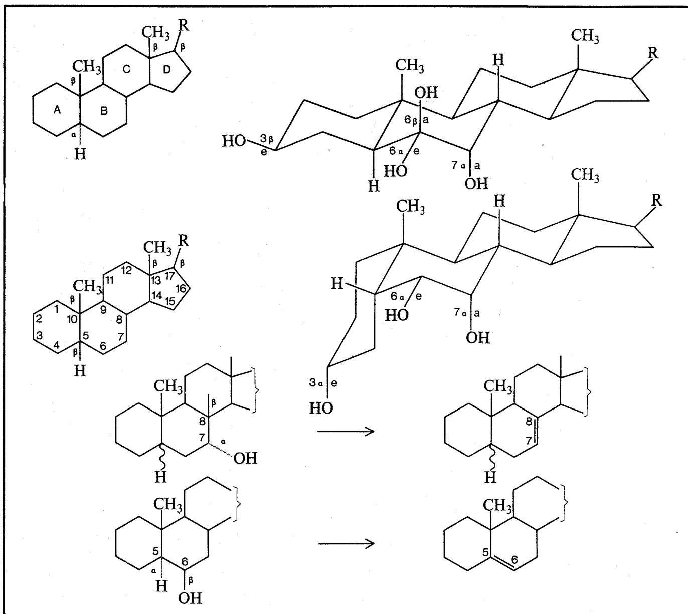
Fig.39 Formule planari e conformazioni dei derivati colestanici (sopra) e coprostanici. Nelle formule planari i legami in nero indicano sostituenti in \beta , i legami in grigio indicano quelli in \alpha , mentre il tratto a serpentina significa che la posizione del sostituito non è determinata. L'analisi conformazionale dà una spiegazione semplice e razionale di molti fenomeni. La maggior stabilità dei sostituenti equatoriali rispetto a quelli assiali ad esempio rende conto del fatto che il 3\beta - e il 6\alpha -idrossicolestano vengono ottenuti in quantità maggiore del 3\alpha e del 6\beta , mentre nella serie coprostanica i composti favoriti sono il 3\alpha e il 6\alpha . La reattività dell'ossidrile 7\alpha è simile nelle due serie, mentre quella dell'ossidrile 6\alpha è nettamente diversa: solo nella serie colestanica si ha infatti una disposizione planare (in conformazione anti ) dell'ossidrile e di un atomo di idrogeno che permette l'eliminazione di acqua e la formazione di un'olefina (formula in basso).
