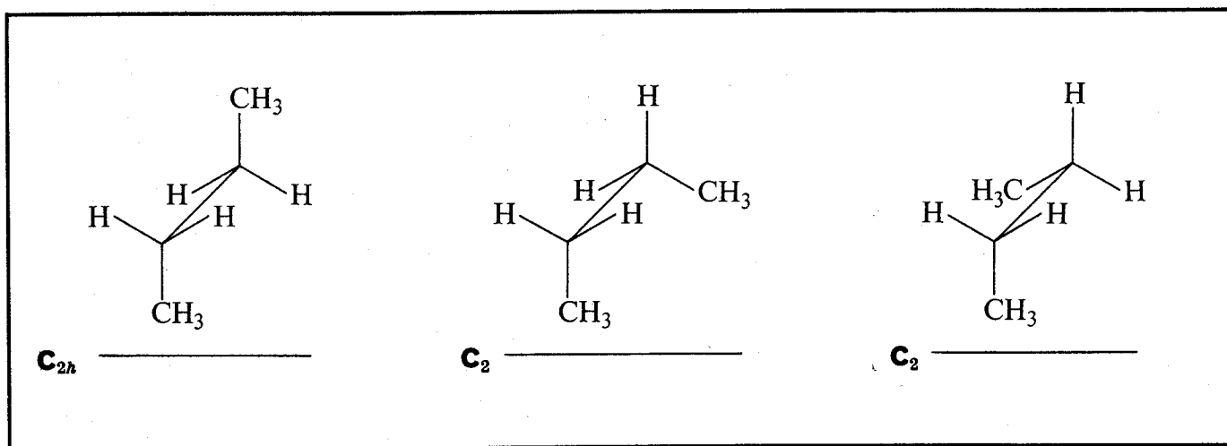
Fig.52 Delle tre conformazioni stabili del butano ( C_4H_{10} ) quella trans , a minor contenuto di energia, è pianosimmetrica (gruppo C_{2h} ) mentre le due conformazioni sghembe sono dissimmetriche (gruppo C_2 ) e antipode tra loro: esse posseggono uguale energia e sono quindi presenti in uguale quantità. Il contributo dell'attività ottica di una forma è bilanciato esattamente da quello dell'altra e inoltre queste due forme si convertono molto rapidamente fra loro e nella forma pianosimmetrica. Il butano è perciò otticamente inattivo.
