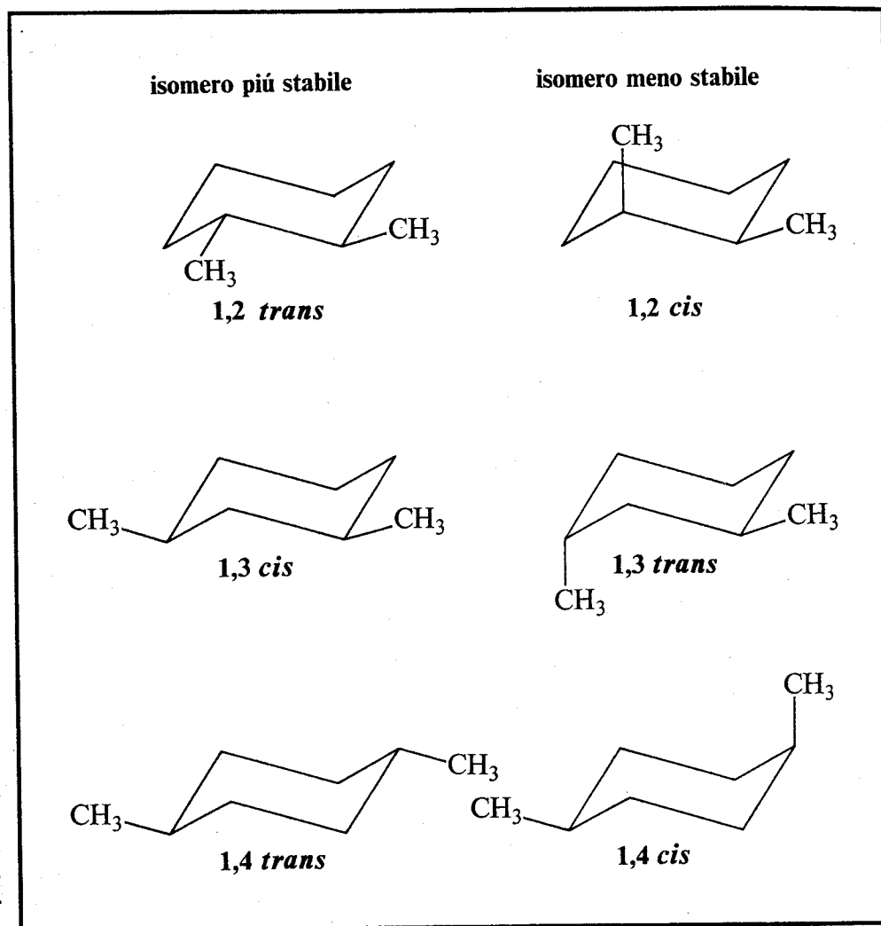
Fig.38 Conformazione dei dimetilcicloesani cis e trans (si confronti con la Fig. 31). Gli isomeri con i due metili in posizione equatoriale sono più stabili di quelli con un sostituito equatoriale e uno assiale. L'esame configurazionale mostra che ai primi corrispondono gli isomeri trans per i cicloesani bisostituiti in 1,2 e in 1,4, e l'isomero cis per il derivato 1,3.
