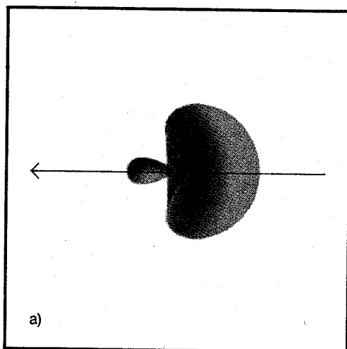
Fig.22 Gli orbitali ibridi hanno una forma a due lobi, uno dei quali è più grande dell'altro (a). I due orbitali ibridi sp hanno la massima espansione in direzioni opposte (angolo di 180^\circ ), i tre orbitali sp^2 sono disposti su un piano a 120^\circ (b), i quattro orbitali sp^3 hanno una disposizione tetraedrica (c).
