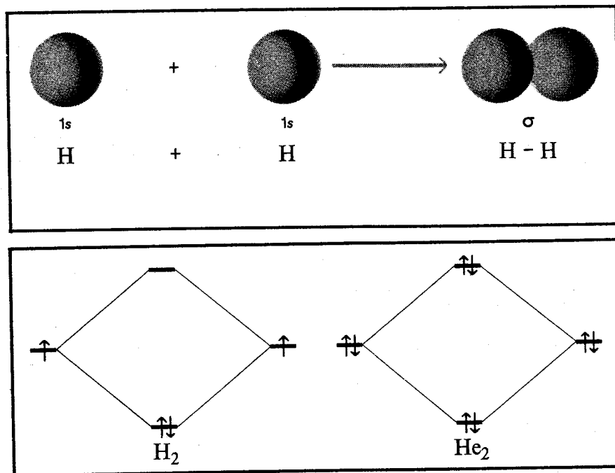
Fig.20 Sopra: combinazione di due orbitali s e formazione di un legame \sigma . La massima densità elettronica è situata sulla congiungente dei due atomi. Sotto: livelli energetici degli orbitali molecolari. L'orbitale a minor energia (in basso) si chiama orbitale di legame, l'altro, orbitale di antilegame. Gli elettroni si dispongono a spin antiparalleli nei diversi orbitali a partire dai livelli energetici più bassi. A sinistra, diagramma energetico di una molecola di idrogeno H_2 e, a destra, quello di una ipotetica molecola di elio He_2 .
