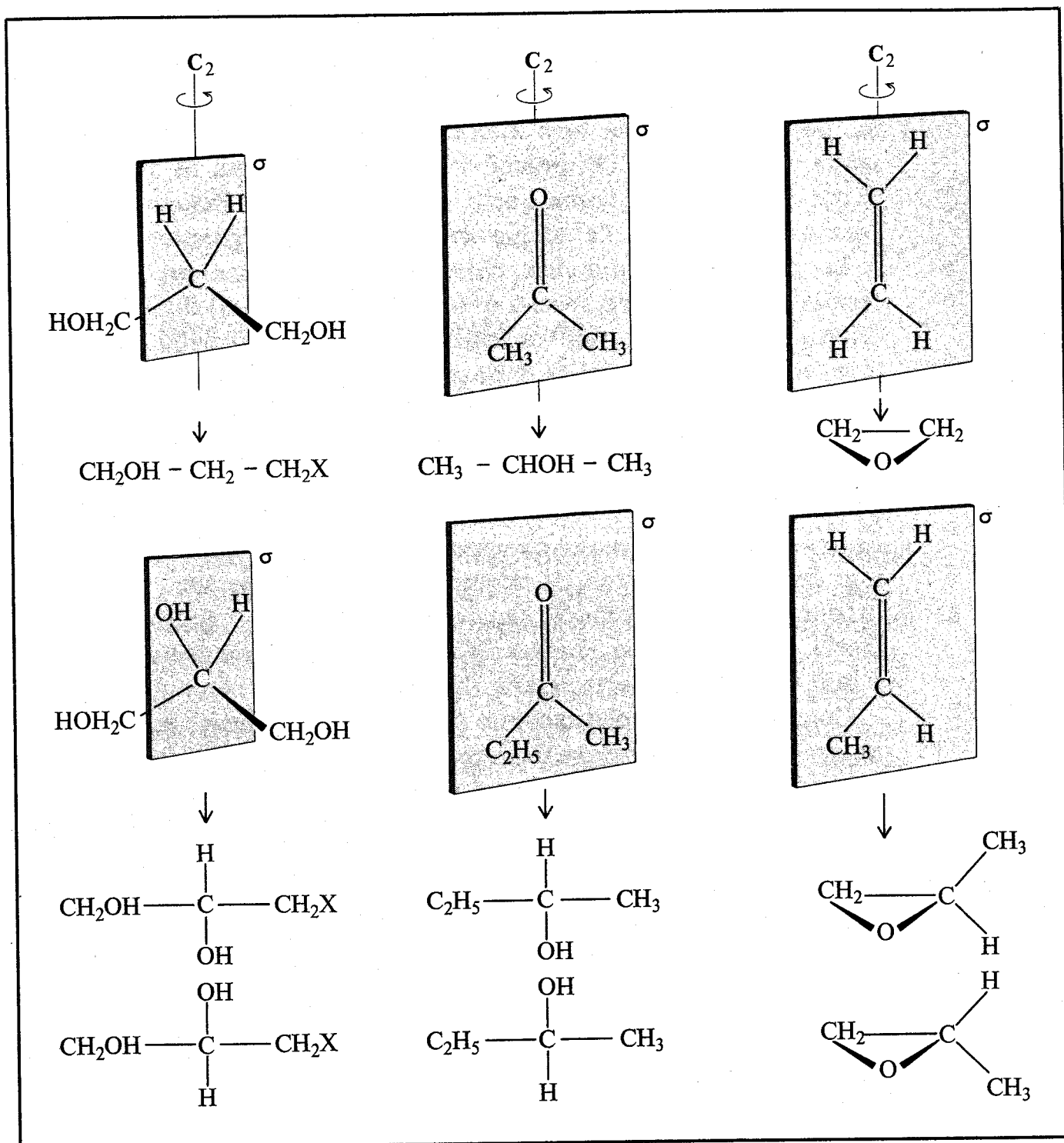
Fig.77 Esempi di molecole prochirali e non. Queste ultime sono caratterizzate dalla presenza di assi di rotazione che collegano i punti reattivi della molecola e li rendono perfettamente equivalenti. Tali punti reattivi possono essere atomi o gruppi di atomi o anche le due opposte facce di un doppio legame. In alto indichiamo alcune molecole che contengono un asse binario e un piano di simmetria; da sinistra, l'1,3-propandiolo, l'acetone e l'etilene. Essi si trasformano ad esempio nel 3-cloropropanolo, nell'alcool iso -propilico e nell'ossido d'etilene, composti che non presentano fenomeni di stereoisomeria. In basso tre esempi di molecole prochirali, in cui è presente il piano di simmetria, ma non l'asse binario. Da sinistra l'1,2,3-propantriolo (o glicerina), il metiletilchetone e il propilene. Con reazioni analoghe a quelle più sopra indicate possono essere convertiti nel 3-cloropropandiolo-1,2, nell'alcool butilico secondario e nell'ossido di propilene. Questi tre composti sono asimmetrici ed esistono in forme enantiomorfe. Con i metodi normali di sintesi i due antipodi sono ottenuti in ugual quantità, ma se si fa agire sulla reazione un fattore di asimmetria si può ottenere una prevalenza più o meno marcata di uno dei due antipodi.
