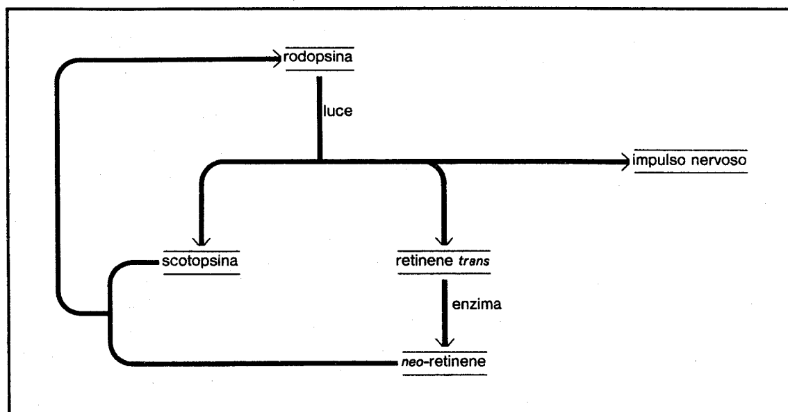
Fig.114 Sotto l'azione della luce la rodopsina si scinde in una proteina (la scotopsina) e nel trans -retinene e contemporaneamente viene emesso uno stimolo nervoso. Il trans -retinene viene poi convertito nel neo -retinene che si ricombina con la proteina per formare la rodopsina. La rigenerazione della rodopsina avviene assai lentamente: è per questa ragione che di notte le luci intense producono fenomeni di abbagliamento.
