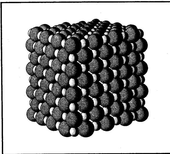
Fig.18 La struttura di un cristallo di sale marino, NaCl o cloruro sodico, è caratterizzata dall'alternanza di ioni \text{Na}^+ e \text{Cl}^- . Gli ioni sono tenuti vicini da forze elettrostatiche. Quando il cloruro sodico viene sciolto nell'acqua, le molecole di questa solvatano gli ioni e di conseguenza diminuiscono fortemente le interazioni fra le cariche opposte.
