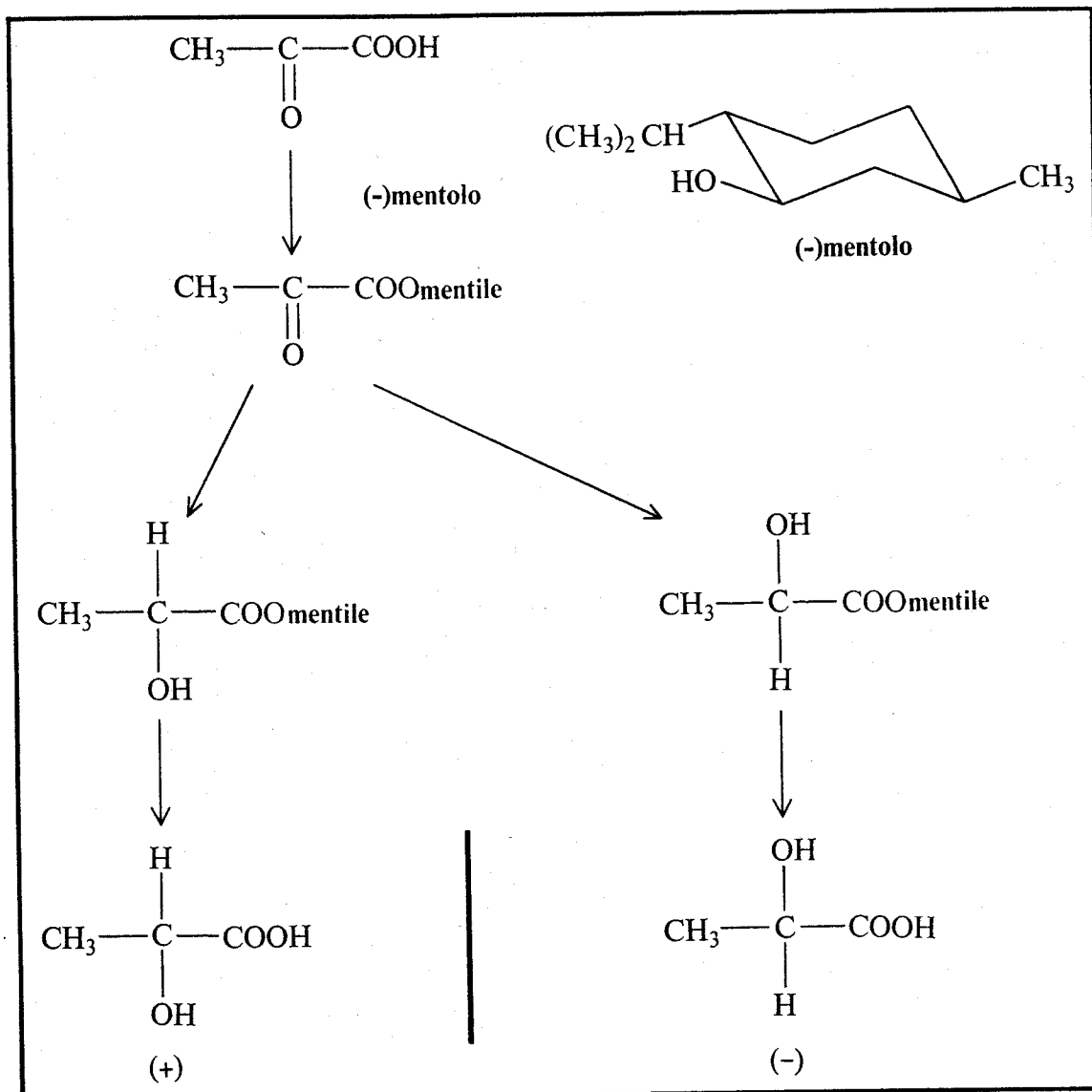
Fig.75 Nella figura precedente abbiamo visto un esempio di induzione asimmetrica intramolecolare. Nella riduzione asimmetrica dell'acido piruvico abbiamo un esempio tipico dell'intervento di un agente asimmetrico ausiliare. La reazione fra l'acido e il (-)-mentolo, un alcool asimmetrico, produce un estere otticamente attivo la cui riduzione dà luogo a quantità non uguali di due esteri diastereoisomeri. L'eliminazione del mentolo dai due esteri conduce all'acido lattico otticamente attivo per la presenza di quantità diverse dei due antipodi.
