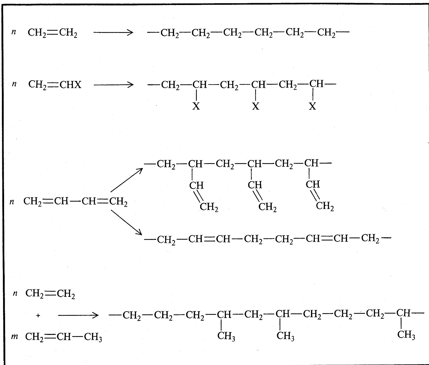
Fig.79 Alcuni esempi di polimerizzazione o poliaddizione, con le formule del monomero e del polimero. Dall'alto: l'etilene, un derivato vinilico generico (se X è un atomo di cloro si ha il cloruro di vinile, se è un metile si ha il propilene, se è un fenile si ha lo stirolo), quindi il butadiene che può polimerizzare in due modi, con un concatenamento 1,2 oppure 1,4. Infine un esempio di copolimerizzazione fra etilene e propilene.
